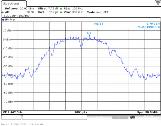
Band Edge NVNT b 2462MHz Ant1 Ref
