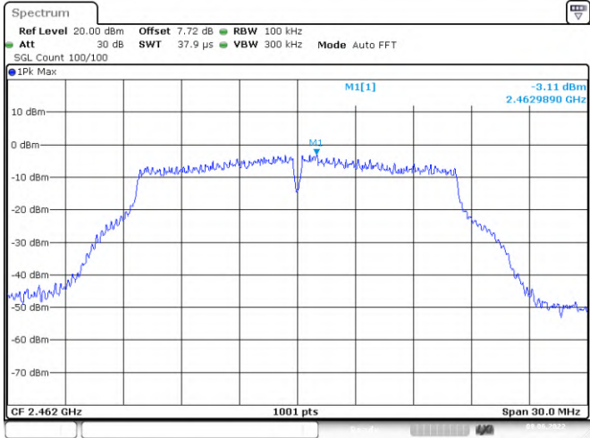
Band Edge NVNT g 2462MHz Ant1 Ref
