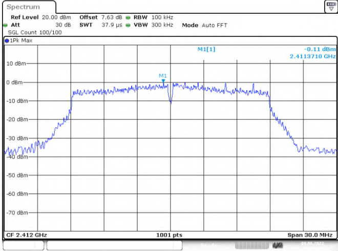
Band Edge NVNT n20 2412MHz Ant1 Ref
