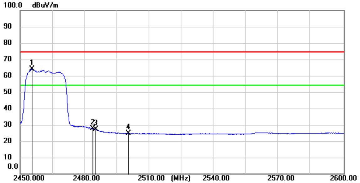
11n(HT20)_TX_CH_11_Vertical_Average
