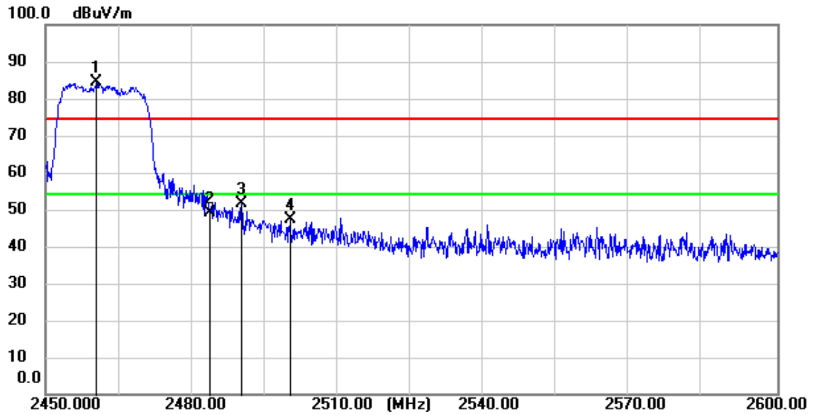
11n(HT20)_TX_CH_11_Vertical_Peak
