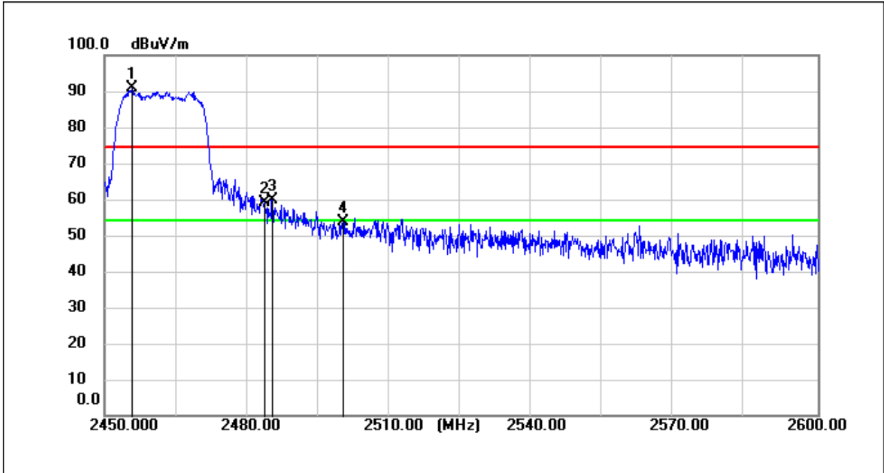
11n(HT20)_TX_CH_11_Horizontal_Peak
