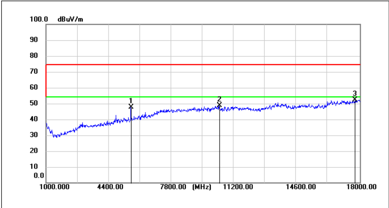
11n(HT20)_TX_CH_11_Vertical
