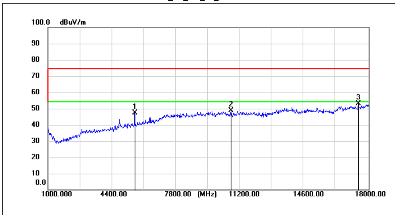
11b_TX_CH_06_Vertical
