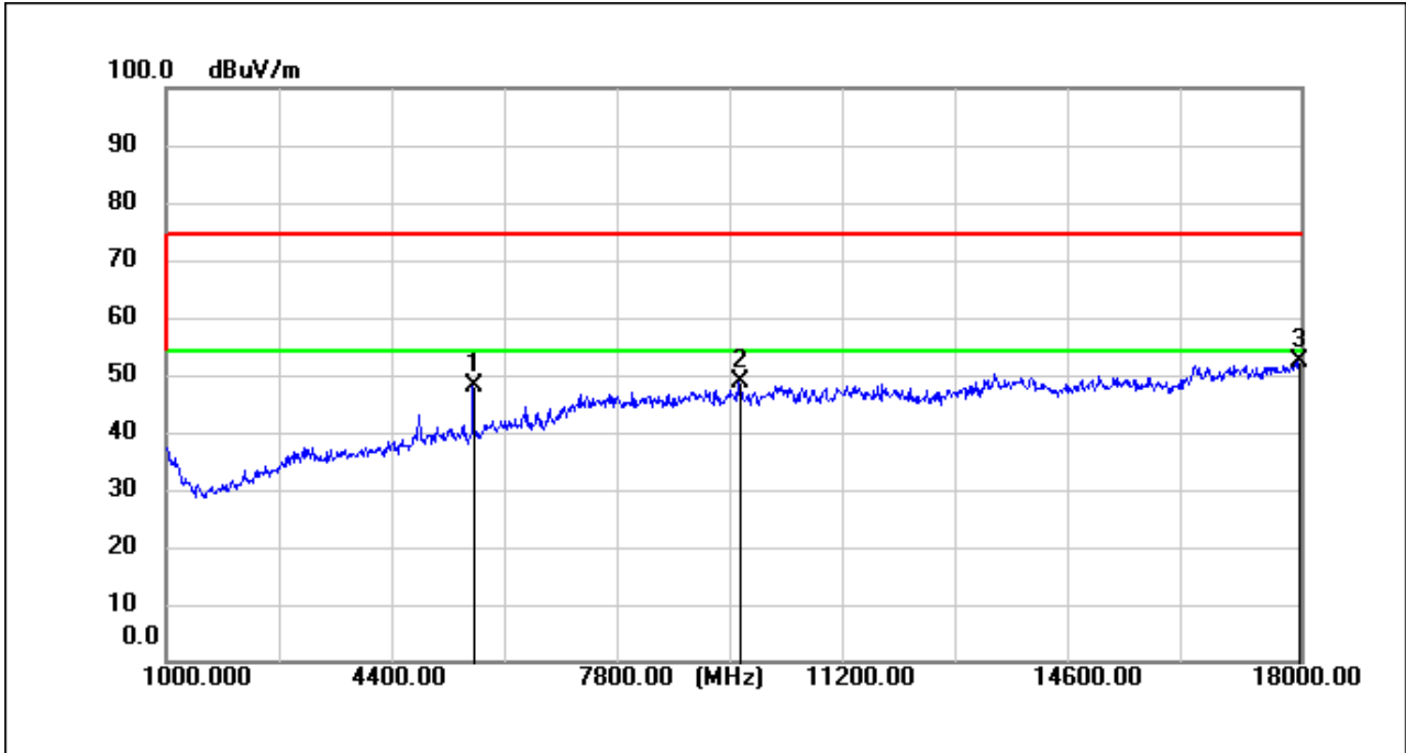
11n(HT20)_TX_CH_06_Vertical
