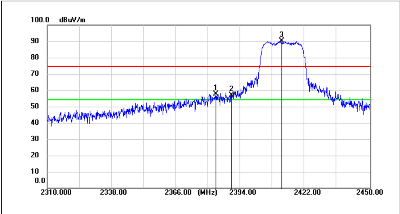
11n(HT20)_TX_CH_01_Horizontal_Peak
