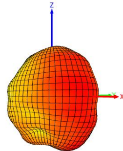
2500MHz
