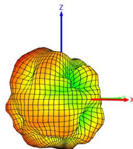
2500MHz
