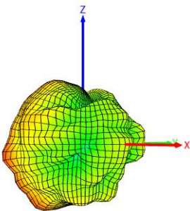
2400MHz
