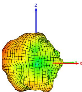
2450MHz
