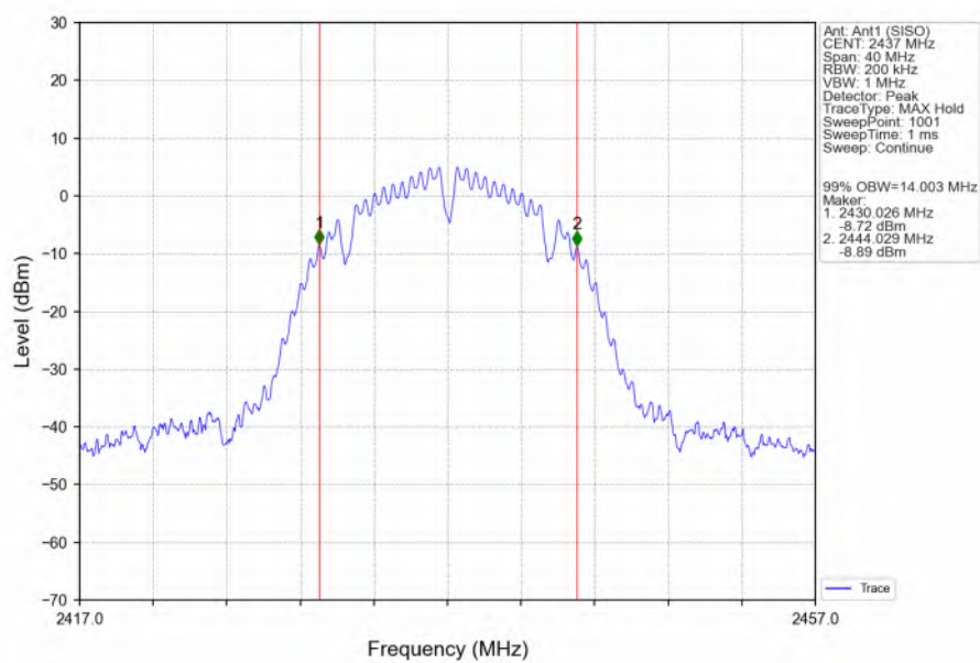
802.11b_MCH_2437MHz_Ant1 (SISO)_NTNV
