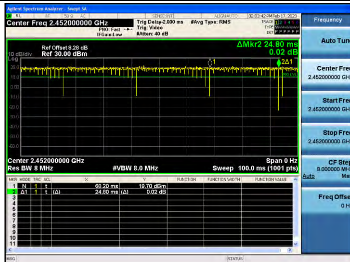
11N40ISO_Ant1_2452
