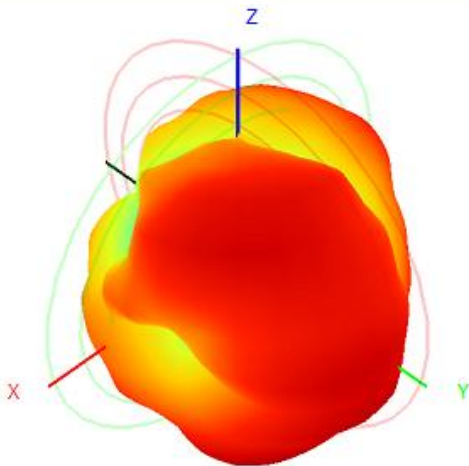
远场方向图
