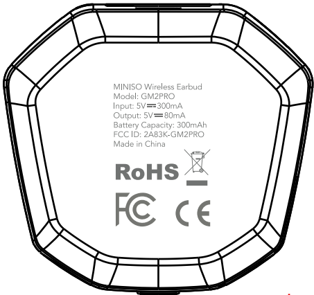
底部
