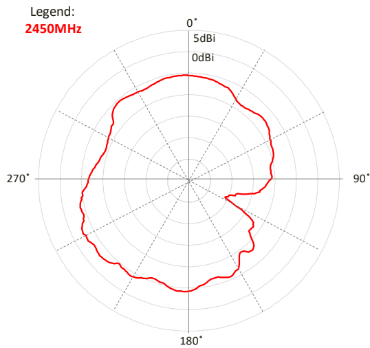
Elevation 1
