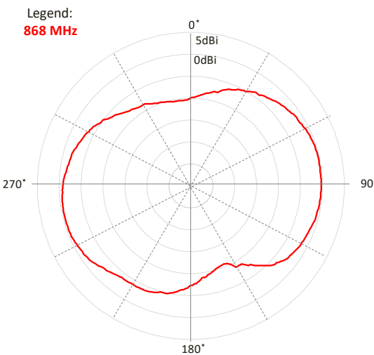
Elevation 2
