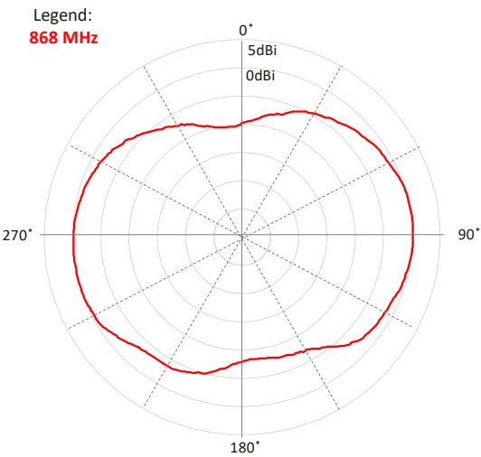
Elevation 1
