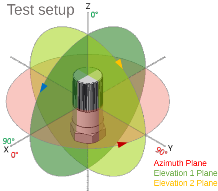
Elevation 1
