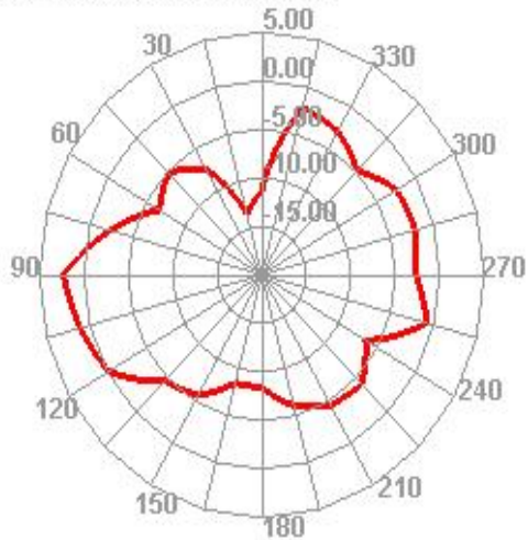
2500.000MHz E2
