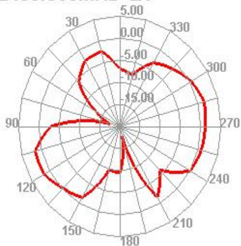
2450.000MHz E1
