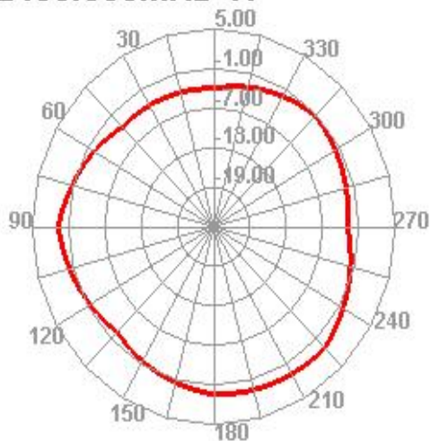
2400.000MHz H
