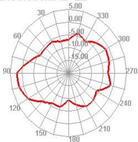
2450.000MHz E2
