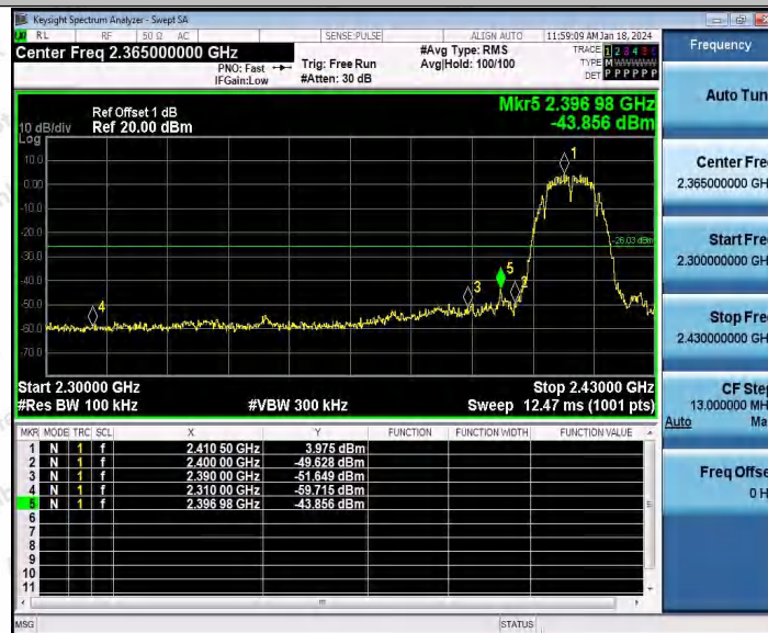
802.11b_Ant1_High_2462
