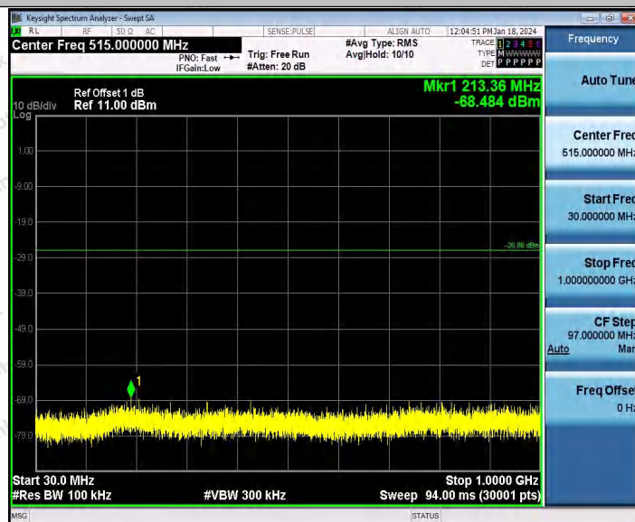
802.11b_Ant1_2437_30~1000
