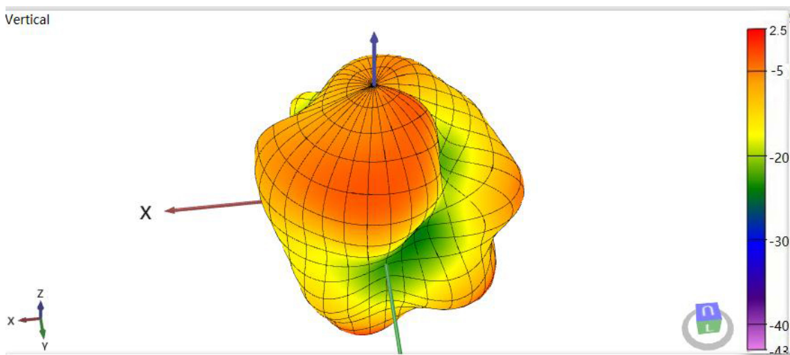
天线 2480MHz 3D-Vertical Pattern
