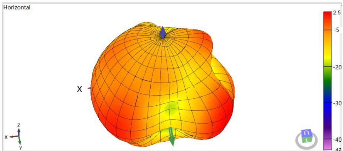
天线 2480MHz 3D-Horizontal Pattern
