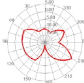
2500.000MHz
