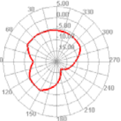
2400.000MHz E2
