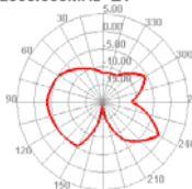
2500.000MHz E1
