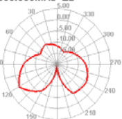
2500.000MHz E2
