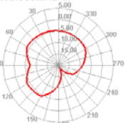
2450.000MHz H
