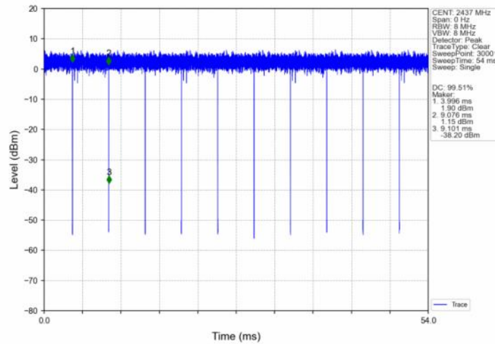
802.11n(HT20)_MCH_2437MHz_Ant1 (SISO)_NTNV
