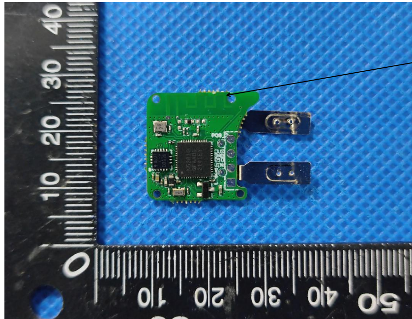
B L E Antenna
