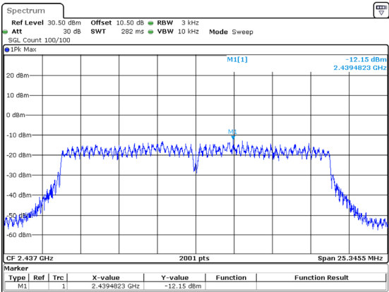
802.11n20_2437MHz
