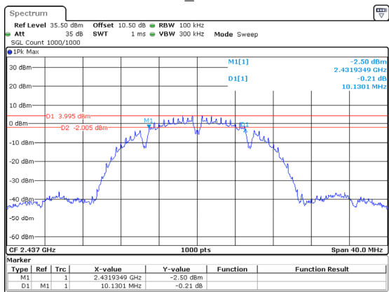
802.11b_2437MHz
