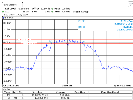
802.11b_2412MHz
