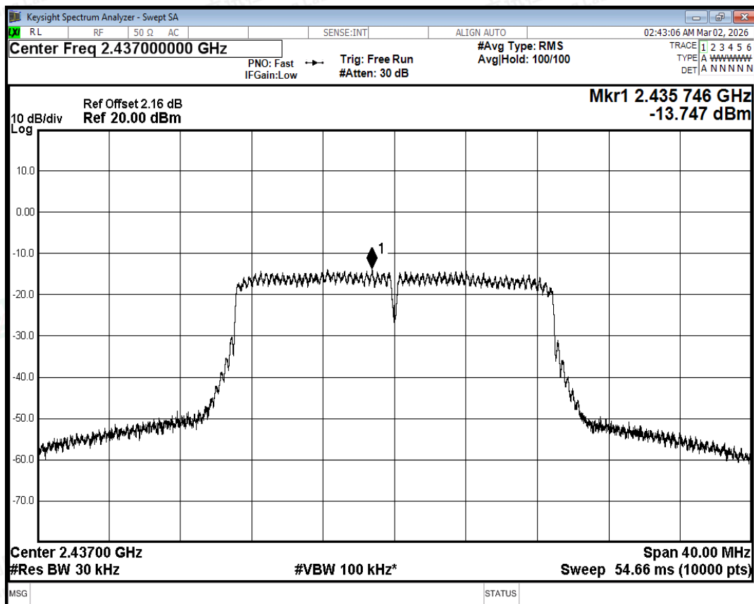
PSD NVNT ax20 2437MHz Ant1
