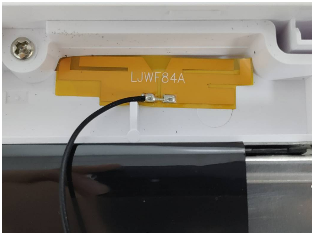
Antenna -BT&WIFI
