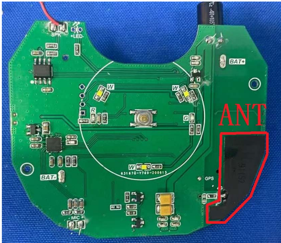
LTE Antenna
