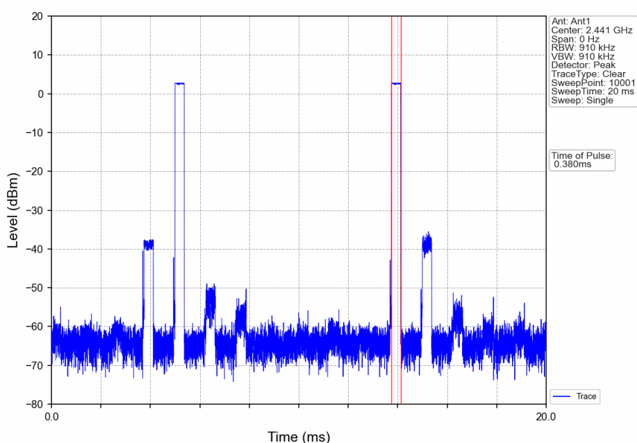
GFSK_DH1_HOPP_Ant1_NTNV
