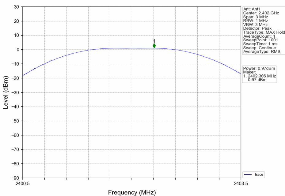
Power NVNT BLE 1M PHY 2402MHz
