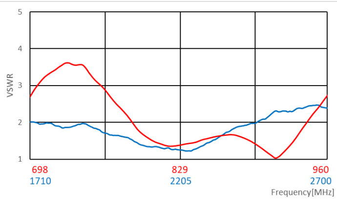
VSWR
