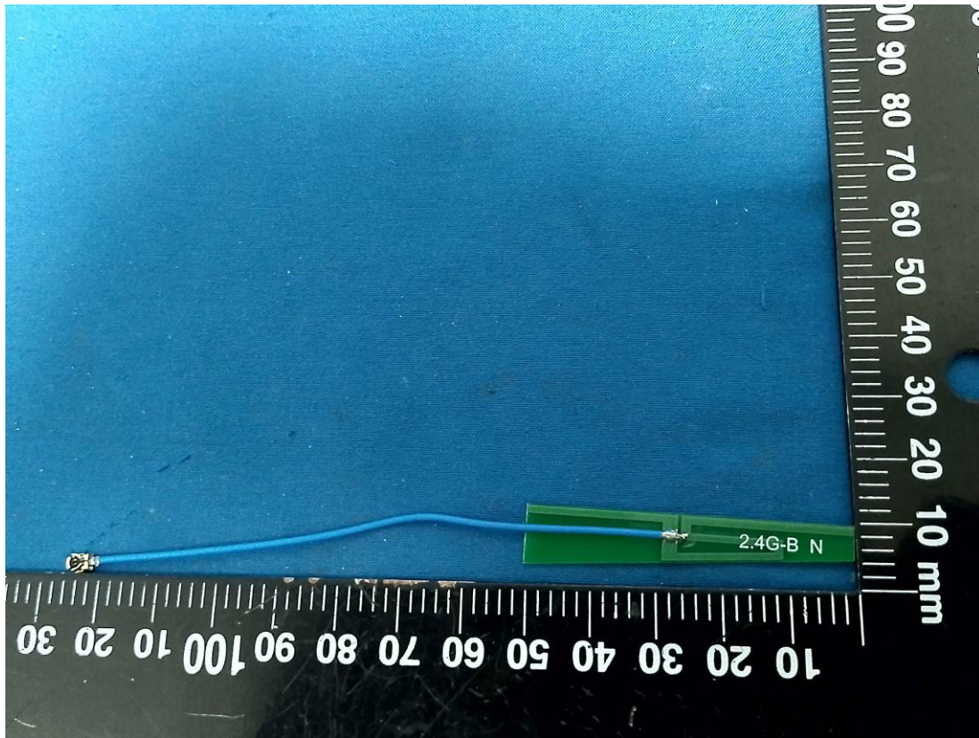
2.4G BLE Antenna
