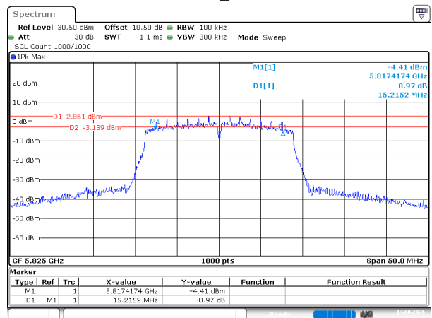
802.11ac20_5825MHz
