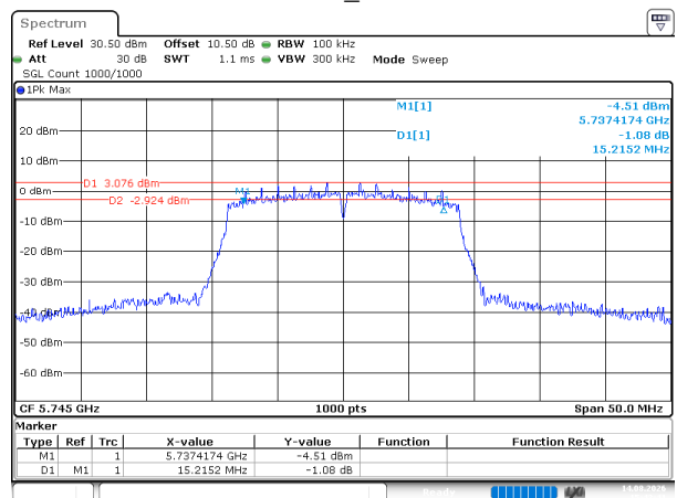
802.11ac20_5745MHz
