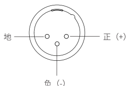
设置正向时端口极性示意
