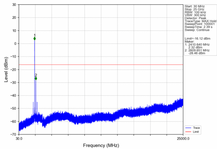
802.11b_LCH_2412MHz_Ant1 (SISO)_NTNV
