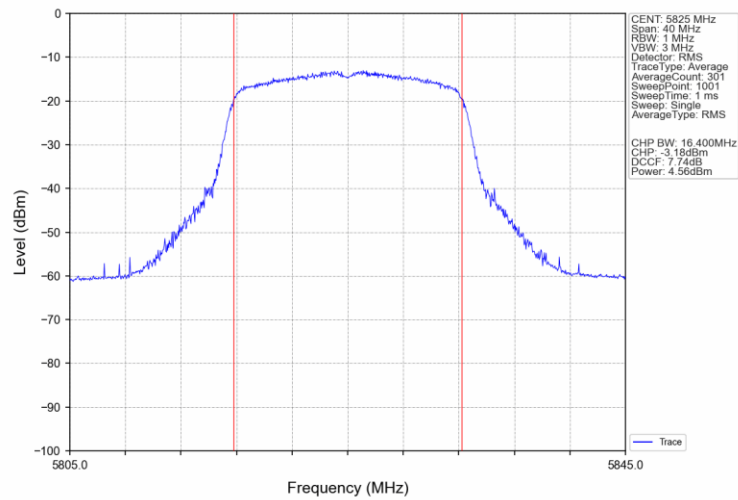
802.11a_HCH_5825MHz_Ant2_NTNV
