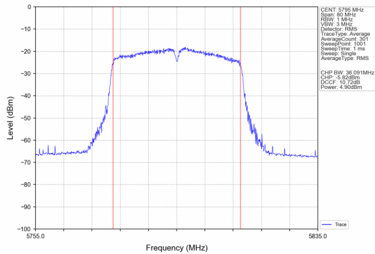
802.11n(HT40)_HCH_5795MHz_Ant2_NTNV
