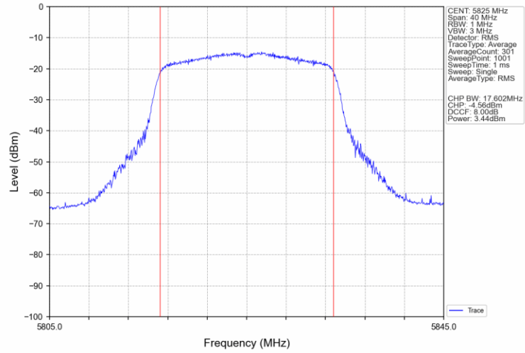
802.11n(HT20)_HCH_5825MHz_Ant2_NTNV
