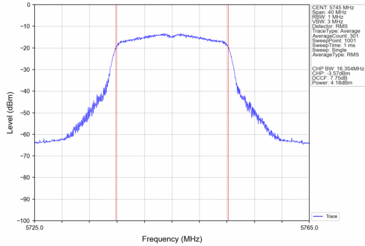
802.11a_LCH_5745MHz_Ant2_NTNV
