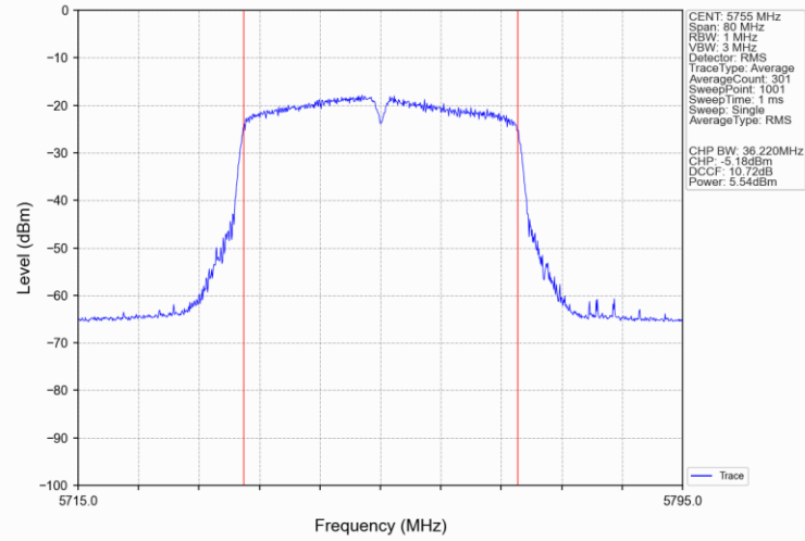
802.11n(HT40)_LCH_5755MHz_Ant2_NTNV
