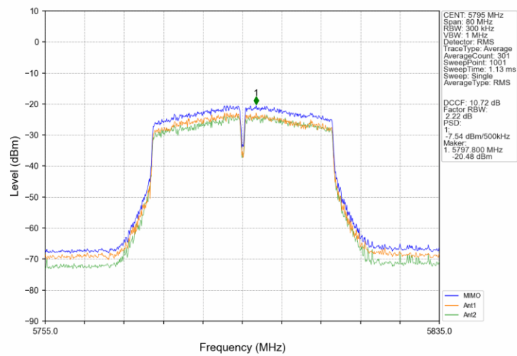
802.11n(HT40)_HCH_5795MHz_MIMO_NTNV
