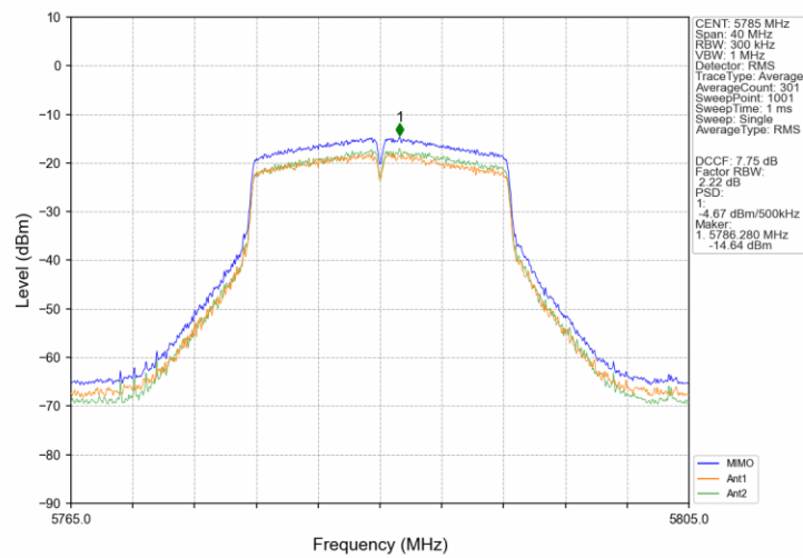
802.11a_MCH_5785MHz_MIMO_NTNV
