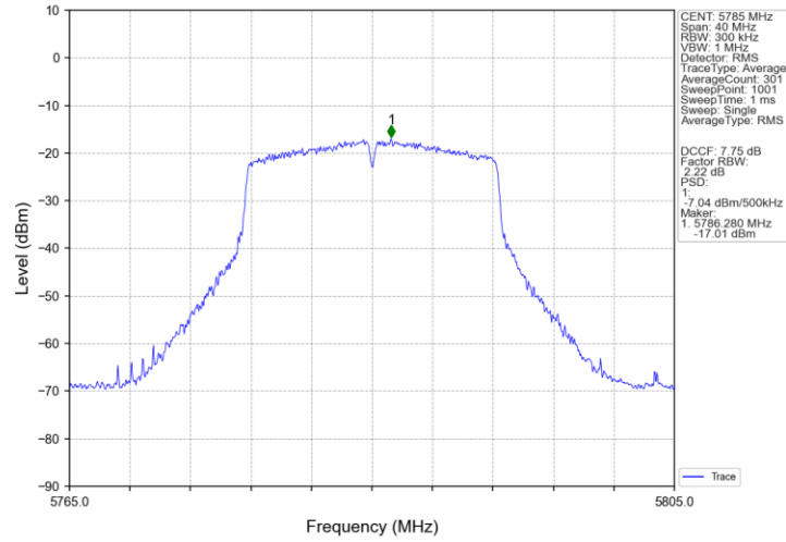
802.11a_MCH_5785MHz_MIMO_NTNV
