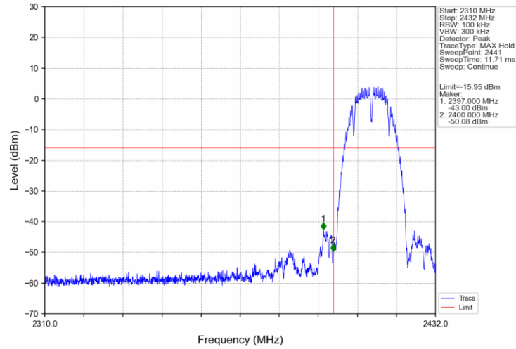
802.11b_LCH_2412MHz_Ant1 (MIMO)_NTNV
