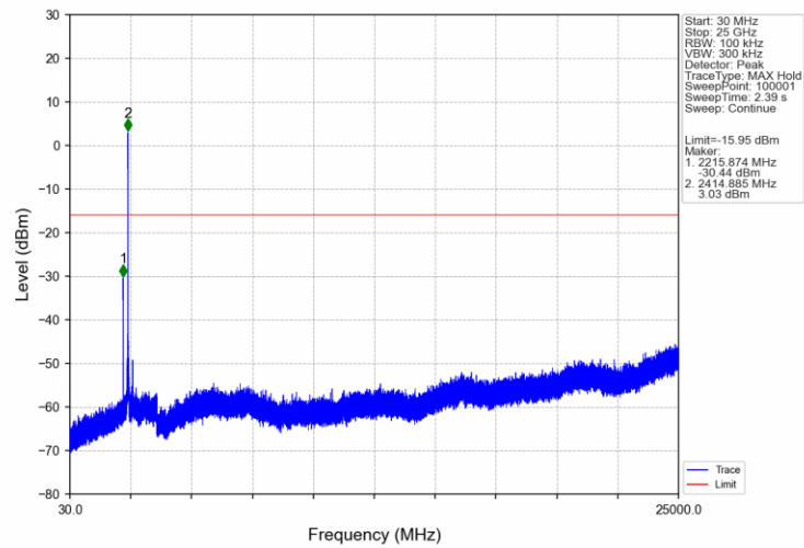
802.11b_LCH_2412MHz_Ant1 (MIMO)_NTNV
