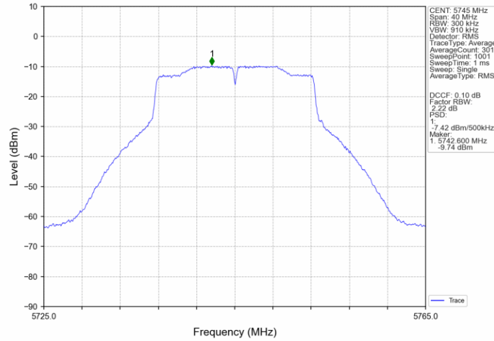
802.11a_LCH_5745MHz_Ant2_NTNV
