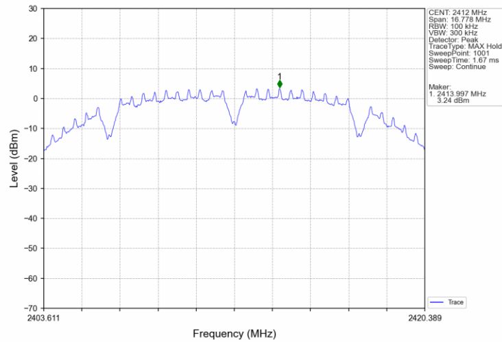
802.11b_LCH_2412MHz_Ant2 (MIMO)_NTNV
