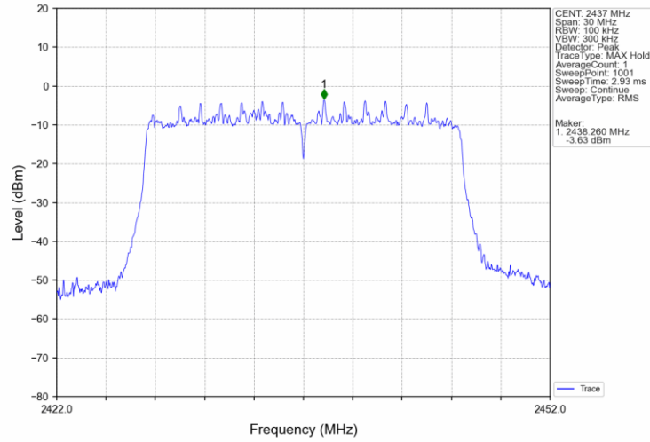
802.11ax(HEW20)_MCH_2437MHz_SU / _MIMO_NTNV
