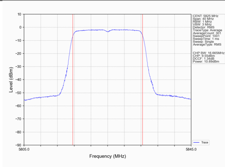
802.11a_HCH_5825MHz_Ant2_NTNV
