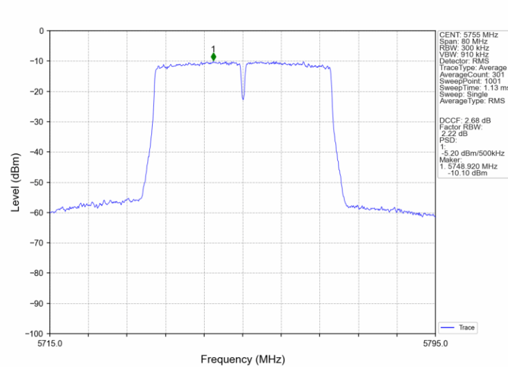
802.11ac(VHT40)_LCH_5755MHz_Ant1_NTNV
