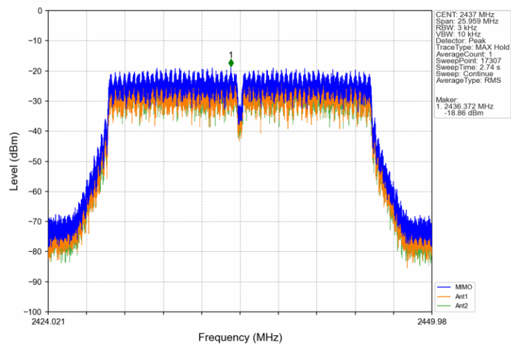
802.11n(HT20)_MCH_2437MHz MIMO NTNV
