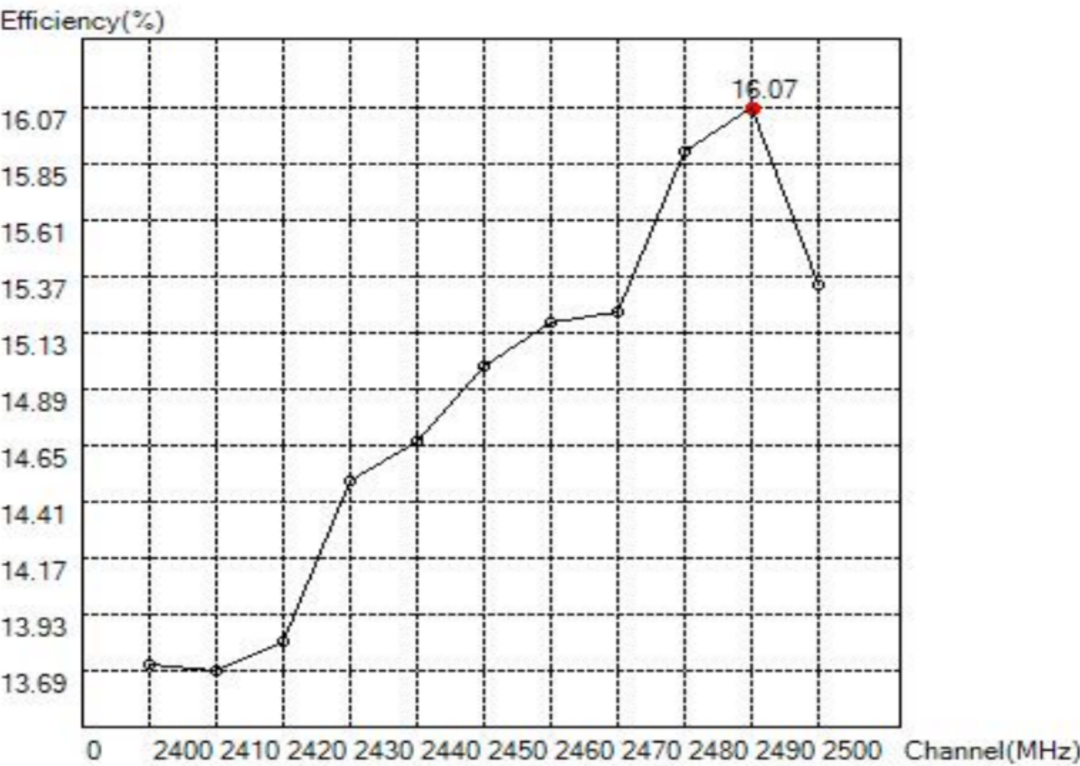
Efficiency-Plane
