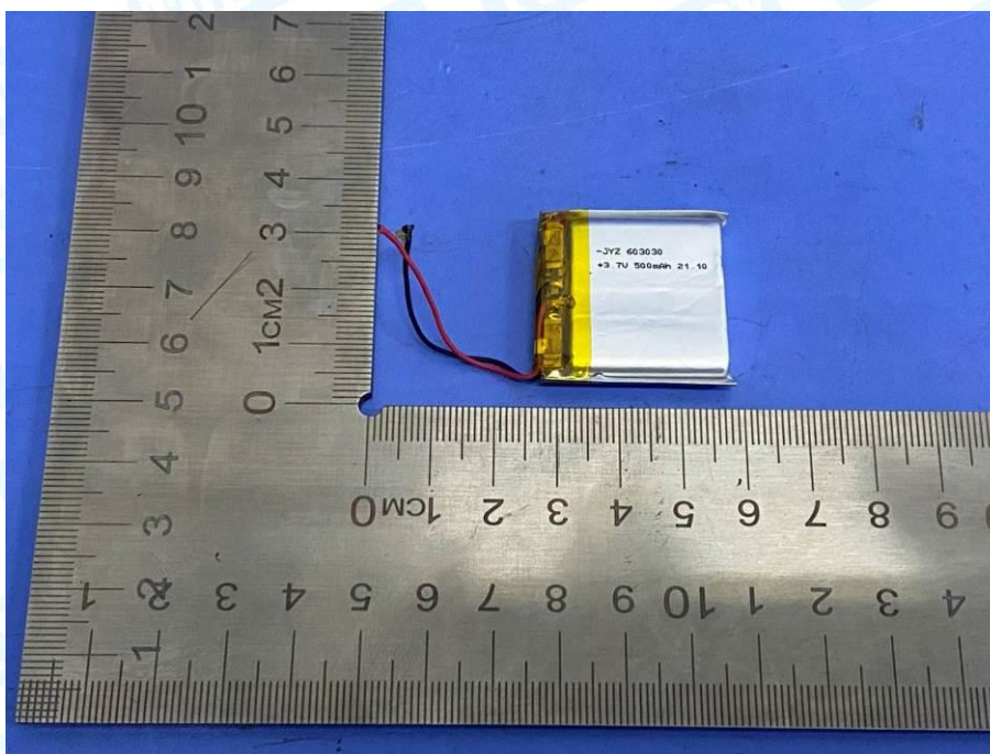
Photo 10 Battery parameters
