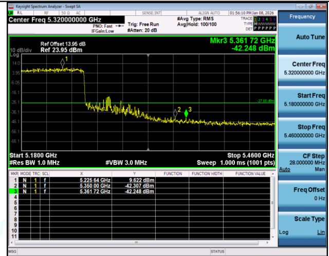
11AX80SISO-Ant1-5210-PASS
