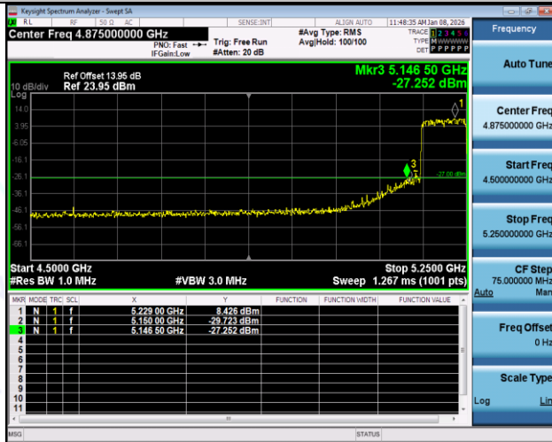
11AC80SISO-Ant1-5210-PASS
