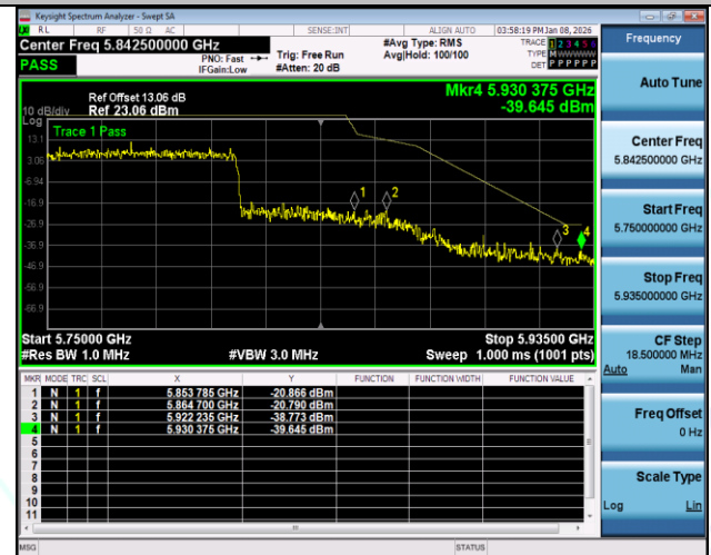
11AX80SISO-Ant1-5775-PASS
