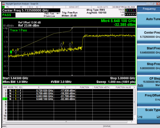
11AX80SISO-Ant1-5775-PASS
