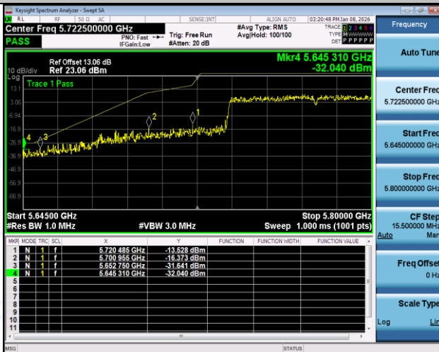
11AC80SISO-Ant1-5775-PASS
