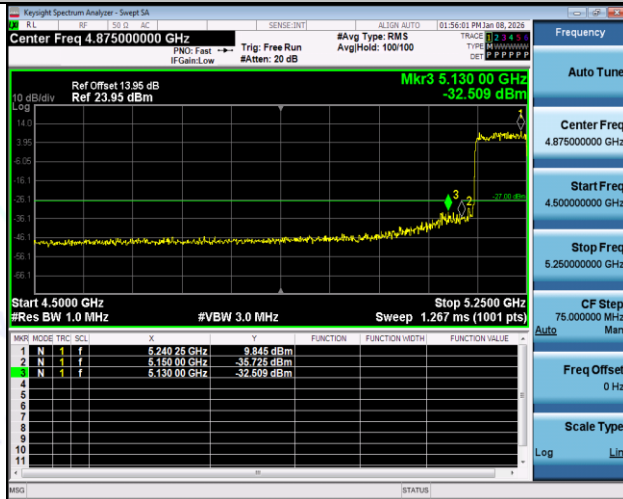
11AX80SISO-Ant1-5210-PASS
