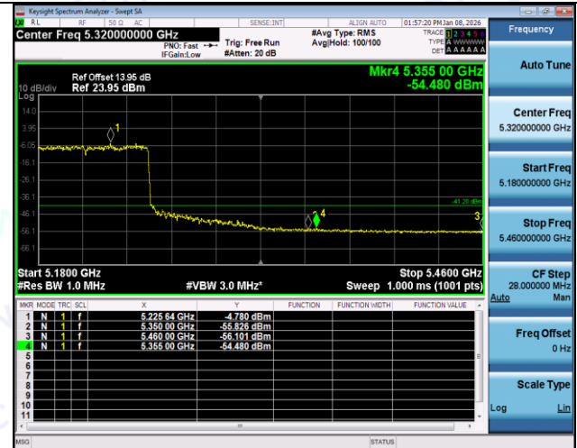
11AX80SISO-Ant1-5210-PASS
