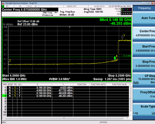
11AX80SISO-Ant1-5210-PASS
