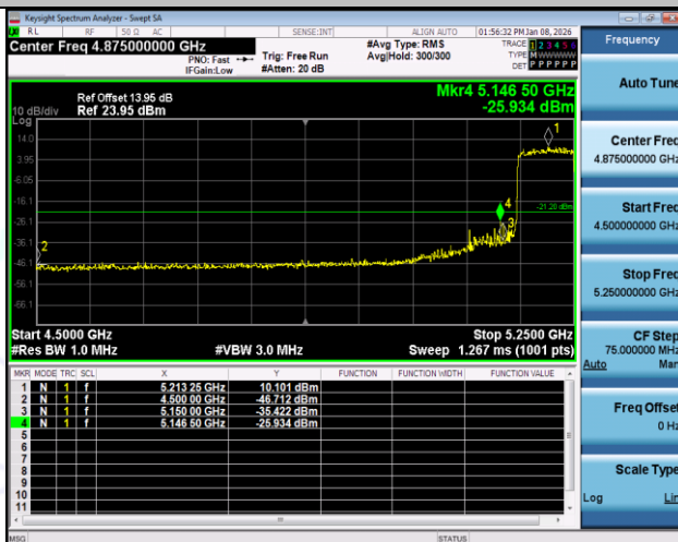
11AX80SISO-Ant1-5210-PASS
