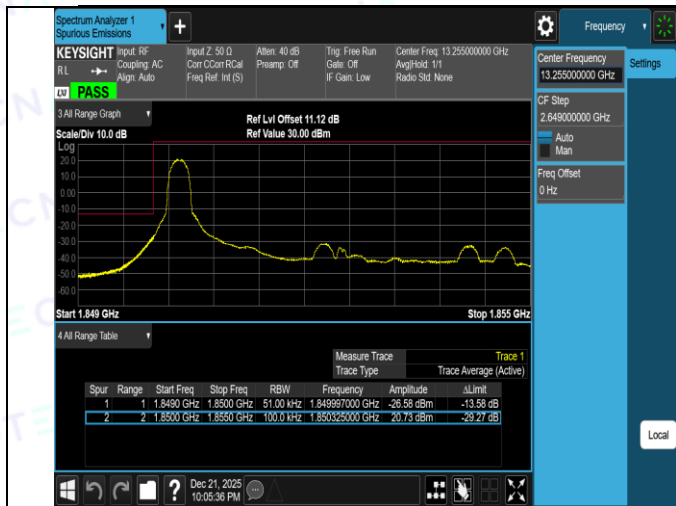
Band2-5MHz-QPSK-18625-25RB#0-PASS
