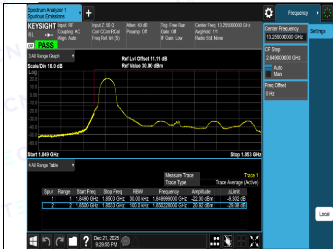
Band2-3MHz-QPSK-18615-15RB#0-PASS
