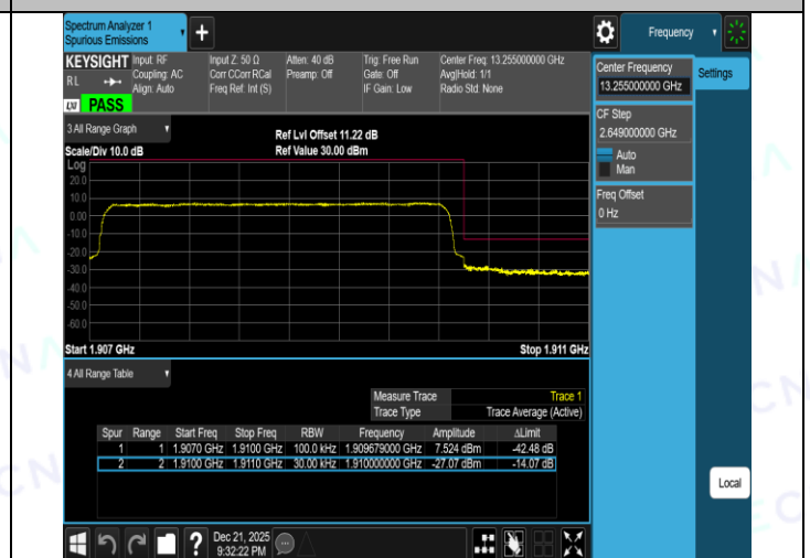
Band2-3MHz-16QAM-18615-1RB#14-PASS
