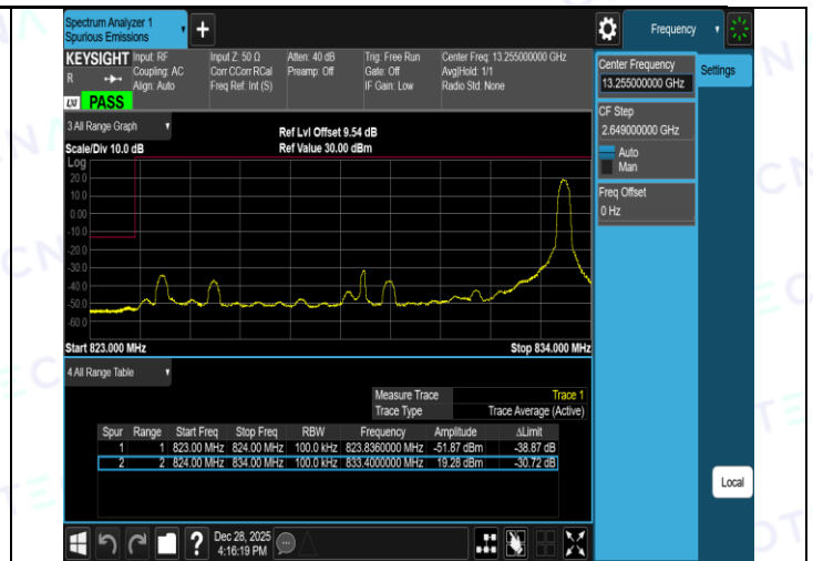
Band26(824-849)-10MHz-QPSK-26990-1RB#0-PASS
