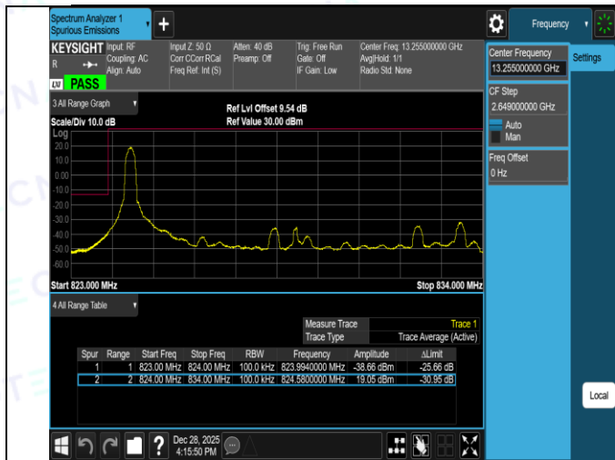
Band26(824-849)-10MHz-QPSK-26840-50RB#0-PASS
