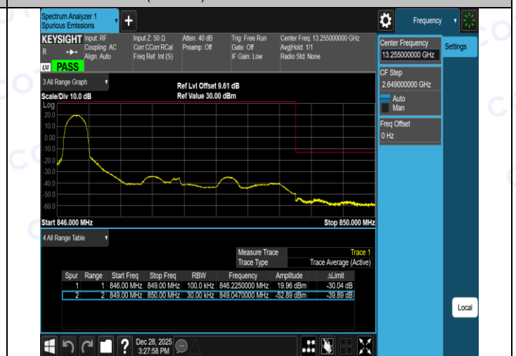
Band26(824-849)-3MHz-QPSK-27025-15RB#0-PASS
