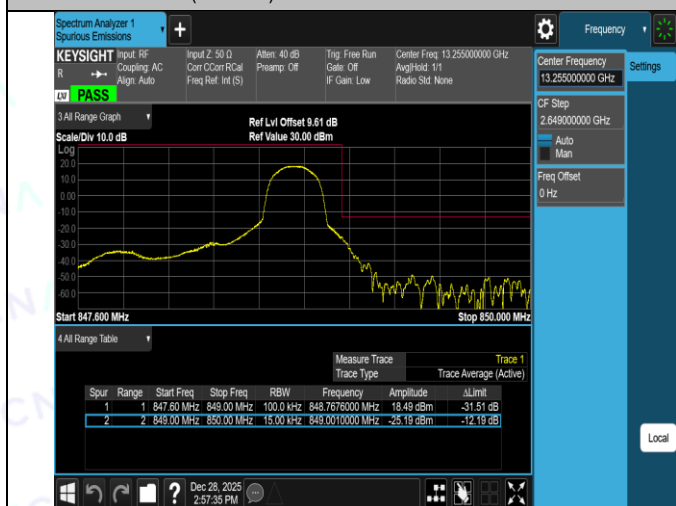
Band26(824-849)-3MHz-QPSK-26805-1RB#0-PASS
