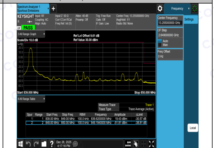
Band26(824-849)-10MHz-QPSK-26990-50RB#0-PASS
