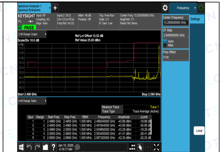
Band38-20MHz-QPSK-38150-1RB#0-PASS
