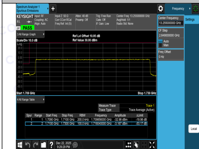
Band66-20MHz-QPSK-132572-1RB#99-PASS
