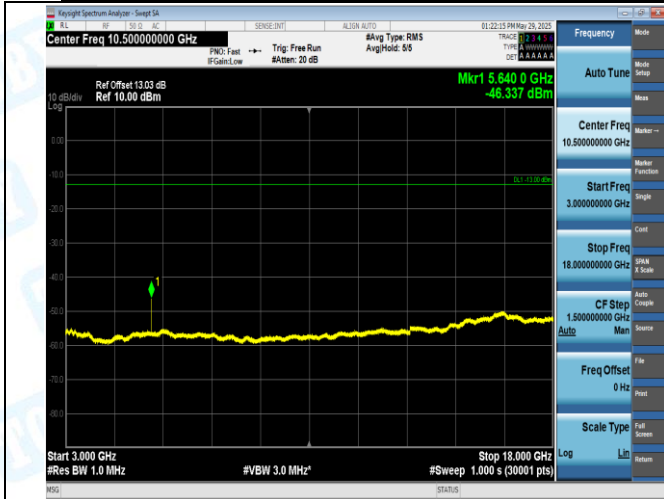
GSM1900-661-0-3000~18000MHz-PASS
