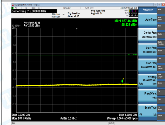
EGPRS1900-512-2-30-1000MHz-PASS
