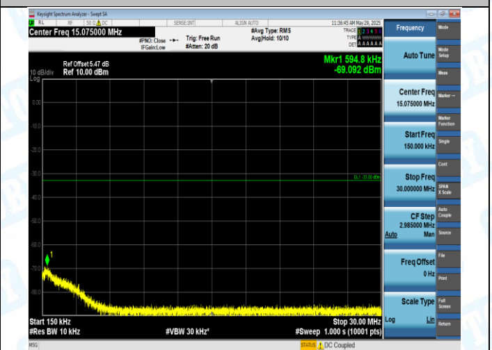
EGPRS1900-810-2-0.15-30MHz-PASS
