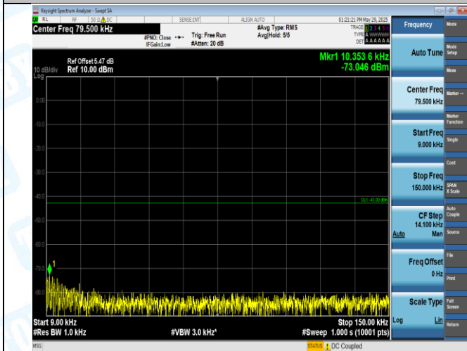
GSM1900-661-0-0.009-0.15MHz-PASS
