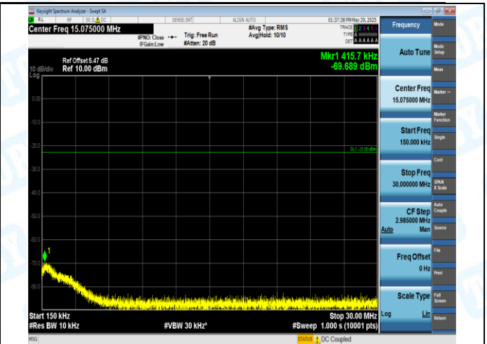
GPRS850-251-5-0.15~30MHz-PASS
