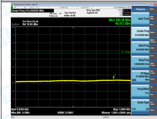
GSM1900-661-0-30-1000MHz-PASS
