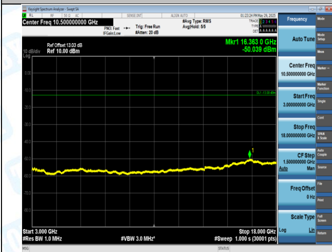
GSM1900-810-0-3000~18000MHz-PASS
