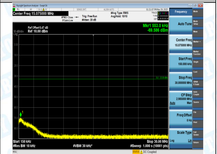
GPRS1900-810-0-0.15~30MHz-PASS
