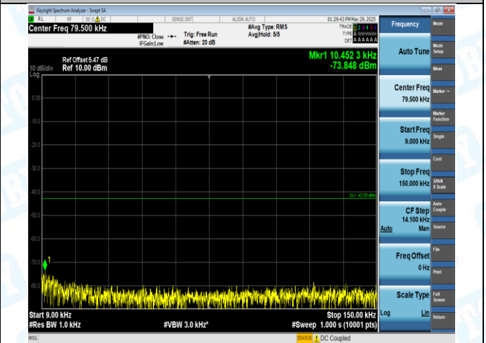
GPRS1900-661-0-0.009-0.15MHz-PASS
