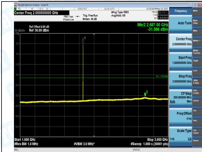
GSM1900-512-0-1000-3000MHz-PASS
