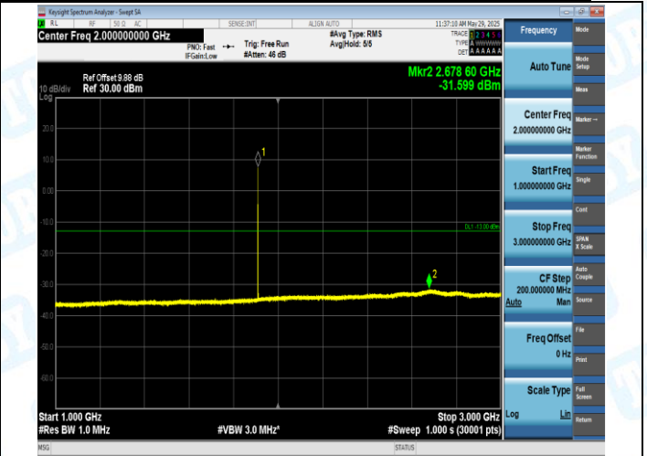
EGPRS1900-810-2-1000~3000MHz-PASS
