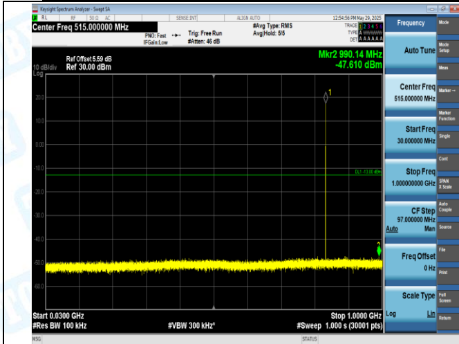
EGPRS850-190-8-30-1000MHz-PASS
