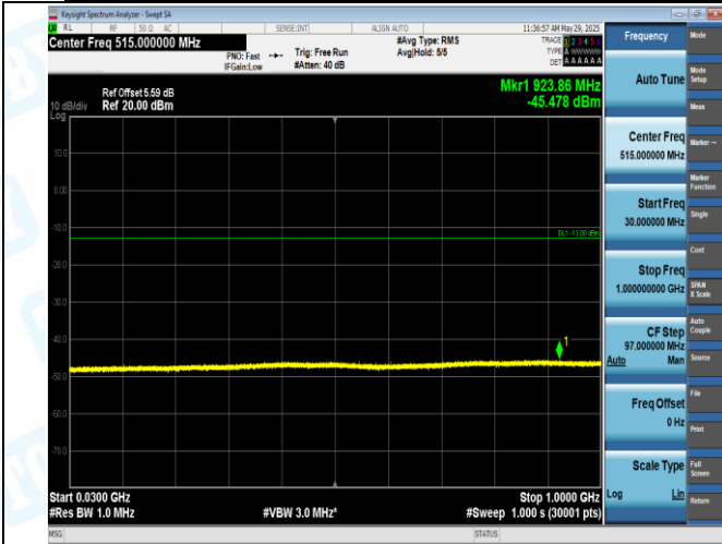
EGPRS1900-810-2-30~1000MHz-PASS
