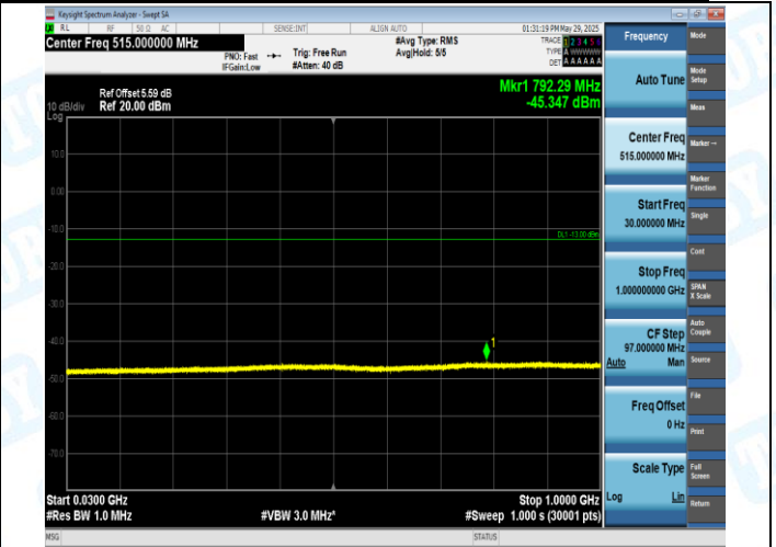
GPRS1900-810-0-30~1000MHz-PASS
