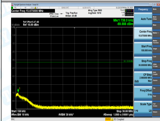
GSM1900-512-0-0.15-30MHz-PASS
