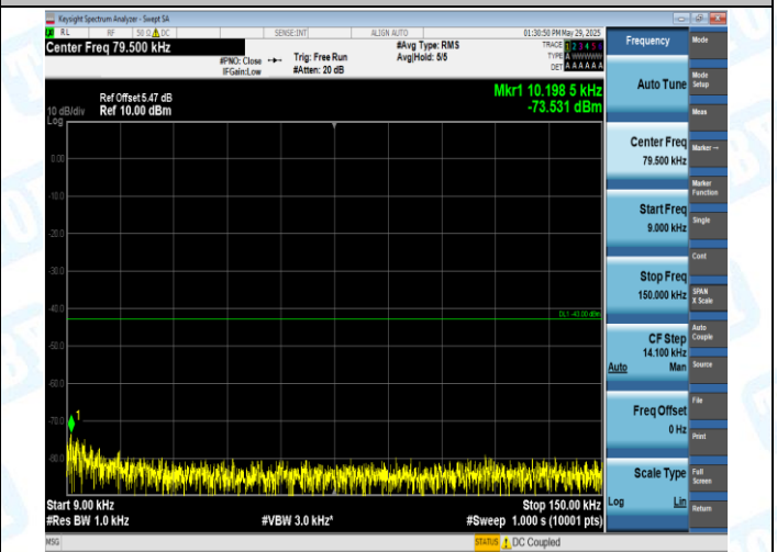
GPRS1900-810-0-0.009~0.15MHz-PASS
