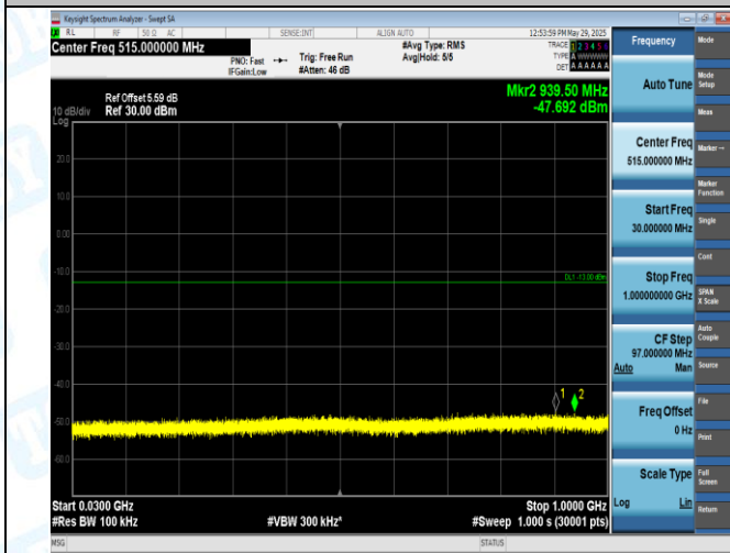
EGPRS850-128-8-30~1000MHz-PASS
