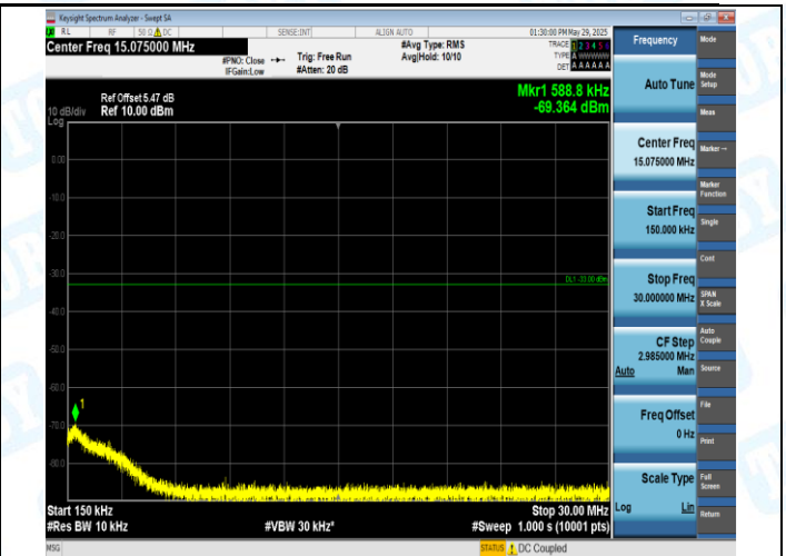
GPRS1900-661-0-0.15-30MHz-PASS
