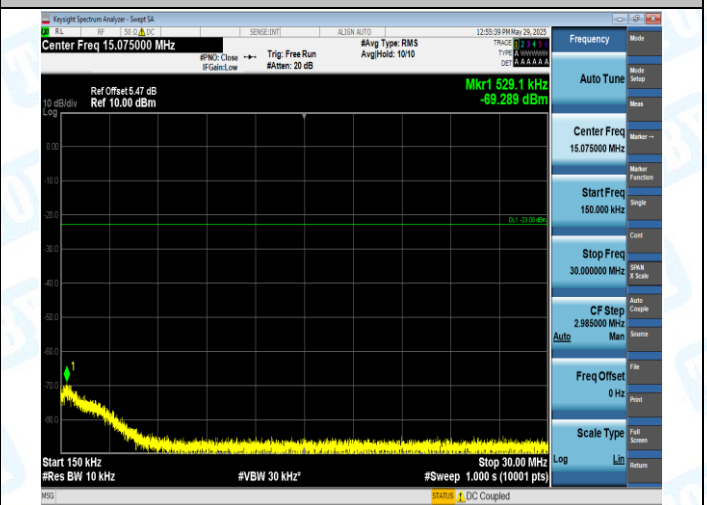
EGPRS850-251-8-0.15-30MHz-PASS
