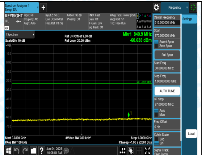
Band2-10MHz-QPSK-18900-1RB#0-30-1000-PASS
