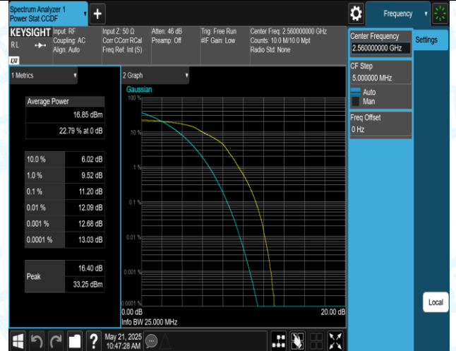
41(2555-2655)-10MHz-16QAM-40290-50RB#0-PASS
