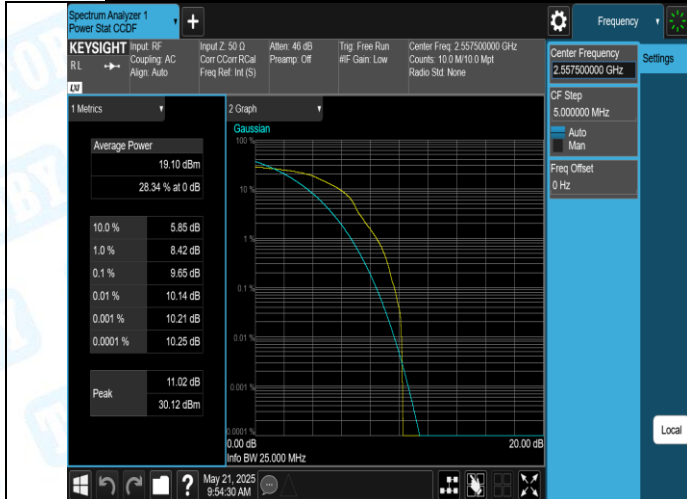
41(2555-2655)-5MHz-16QAM-40265-1RB#0-PASS
