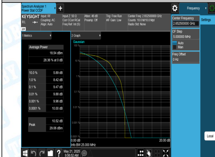
41(2555-2655)-5MHz-16QAM-41215-1RB#0-PASS
