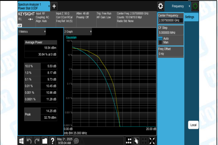
41(2555-2655)-5MHz-16QAM-40265-25RB#0-PASS
