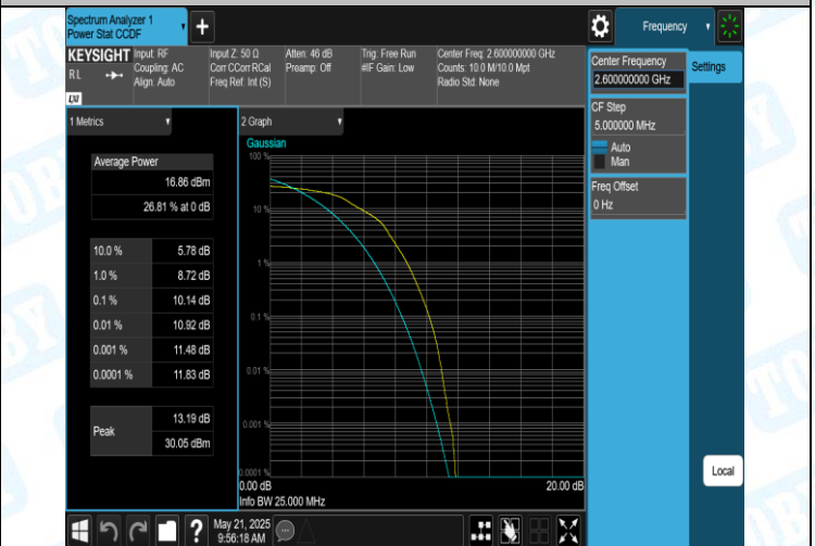
41(2555-2655)-5MHz-16QAM-40690-25RB#0-PASS
