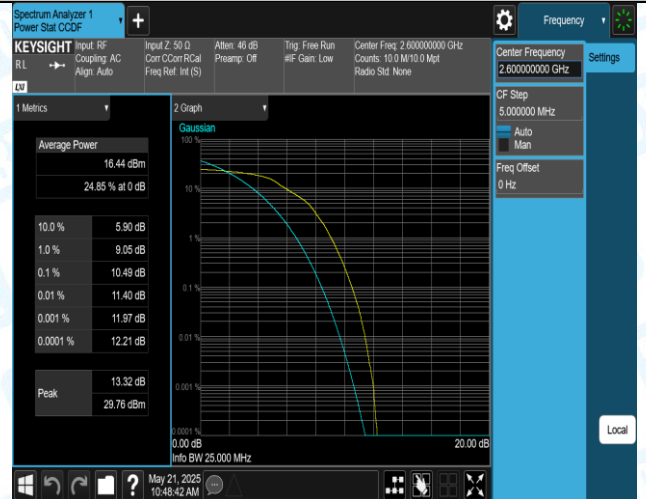
41(2555-2655)-10MHz-16QAM-40690-50RB#0-PASS
