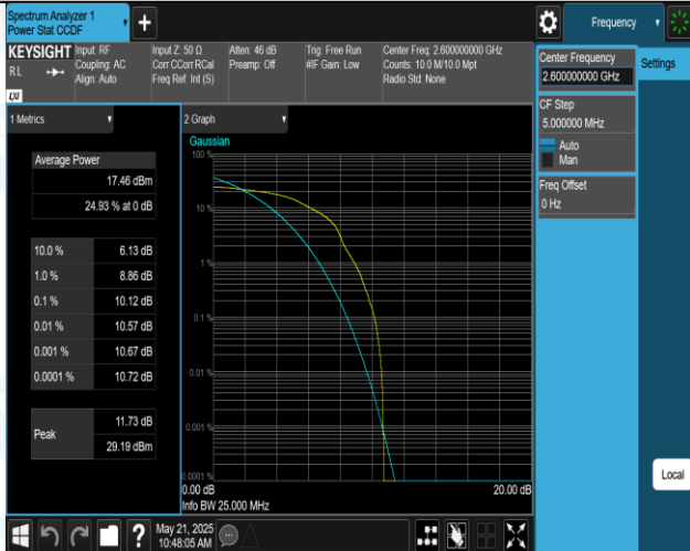
41(2555-2655)-10MHz-16QAM-40690-1RB#0-PASS
