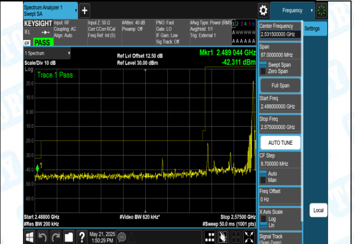
41(2555-2655)-20MHz-16QAM-40340-1RB#99-PASS
