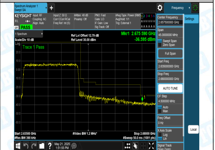
41(2555-2655)-20MHz-16QAM-41140-100RB#0-PASS
