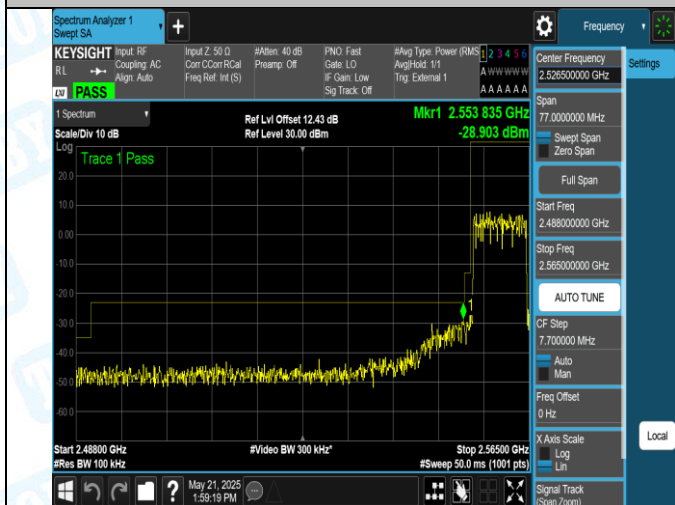
41(2555-2655)-10MHz-QPSK-40290-50RB#0-PASS
