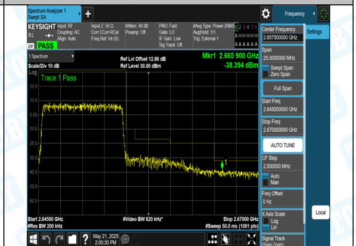
41(2555-2655)-10MHz-16QAM-41190-50RB#0-PASS
