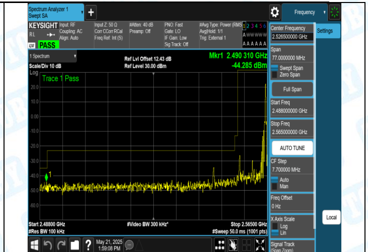
41(2555-2655)-10MHz-16QAM-40290-1RB#49-PASS
