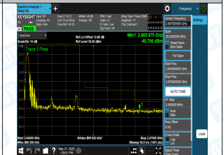
41(2555-2655)-10MHz-16QAM-41190-1RB#0-PASS
