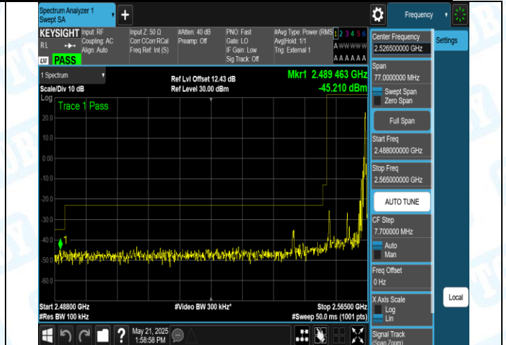
41(2555-2655)-10MHz-QPSK-40290-1RB#49-PASS
