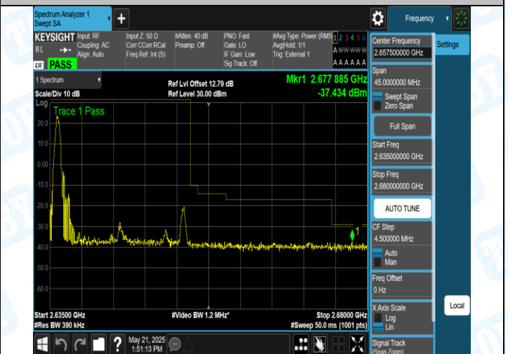
41(2555-2655)-20MHz-16QAM-41140-1RB#0-PASS
