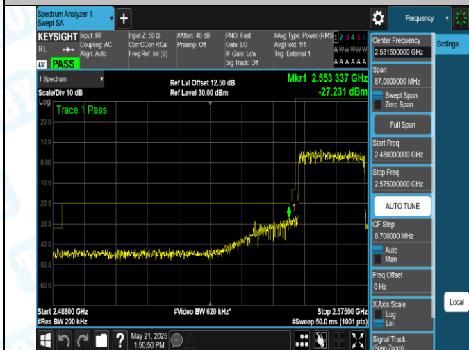
41(2555-2655)-20MHz-16QAM-40340-100RB#0-PASS
