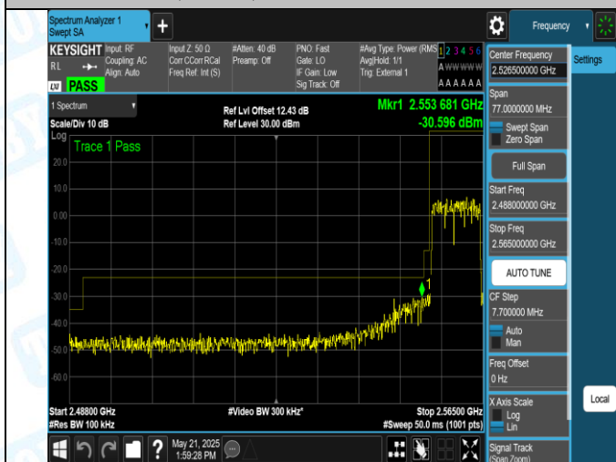
41(2555-2655)-10MHz-16QAM-40290-50RB#0-PASS
