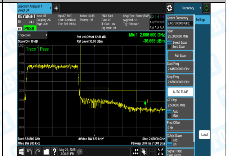
41(2555-2655)-10MHz-QPSK-41190-50RB#0-PASS
