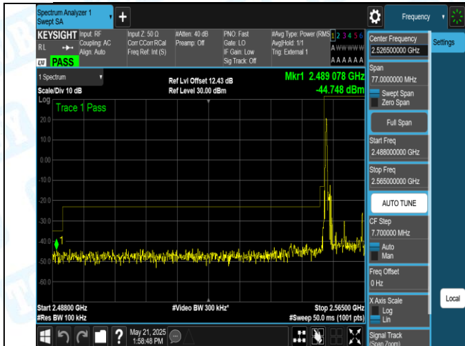
41(2555-2655)-10MHz-16QAM-40290-1RB#0-PASS
