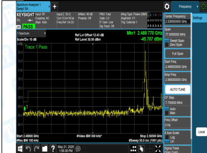
41(2555-2655)-10MHz-QPSK-40290-1RB#0-PASS
