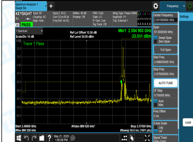
41(2555-2655)-20MHz-16QAM-40340-1RB#0-PASS
