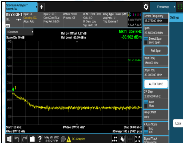
41(2555-2655)-10MHz-QPSK-40690-1RB#0-0.15~30-PASS
