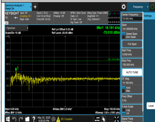
41(2555-2655)-10MHz-QPSK-41190-1RB#0-0.009~0.15-PASS
