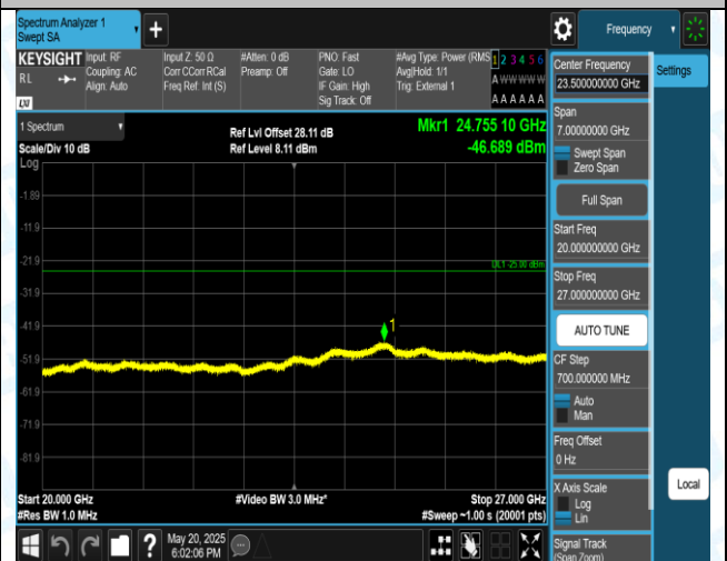
41(2555-2655)-10MHz-QPSK-40690-1RB#0-20000~27000-PASS
