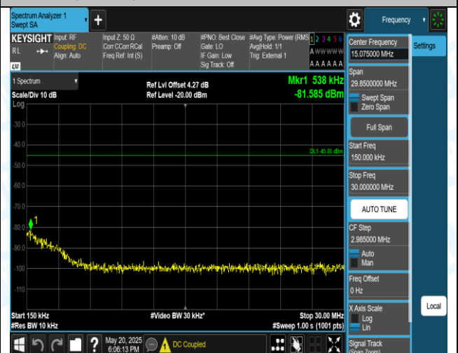
41(2555-2655)-10MHz-QPSK-41190-1RB#0-0.15~30-PASS
