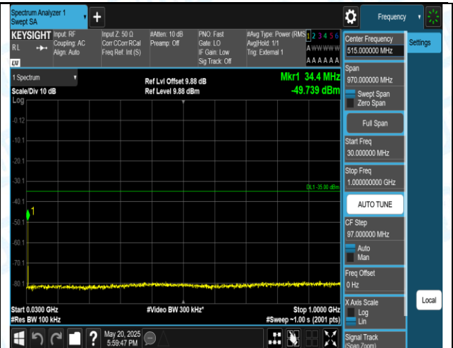
41(2555-2655)-10MHz-QPSK-40690-1RB#0-30~1000-PASS
