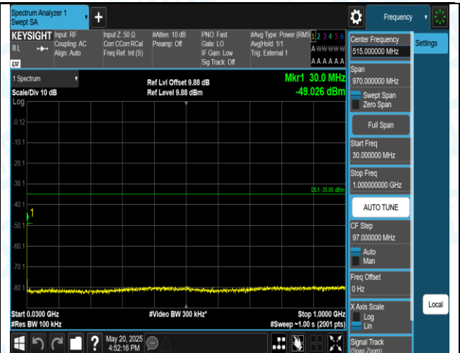
41(2555-2655)-20MHz-QPSK-40690-1RB#0-30~1000-PASS
