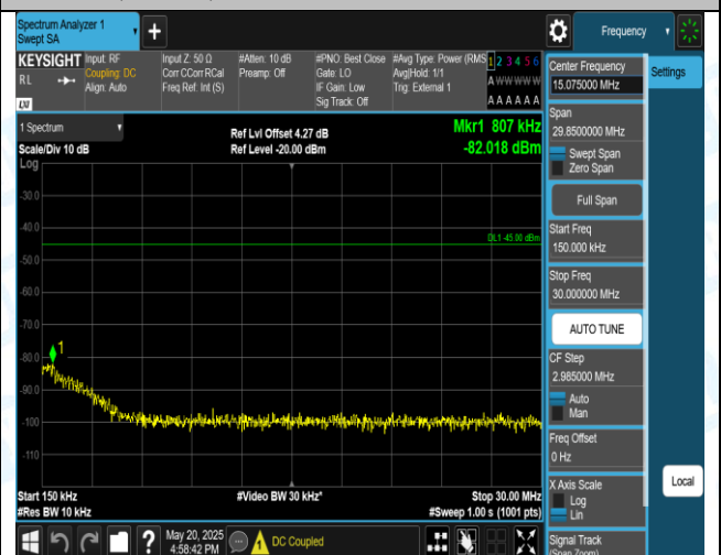
41(2555-2655)-20MHz-QPSK-41140-1RB#0-0.15~30-PASS
