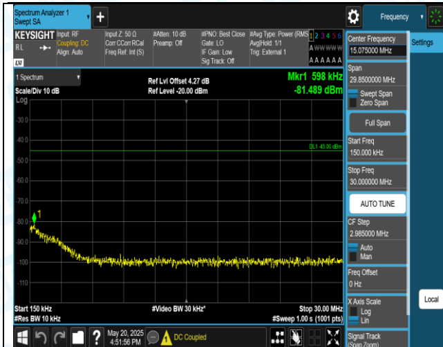
41(2555-2655)-20MHz-QPSK-40690-1RB#0-0.15~30-PASS
