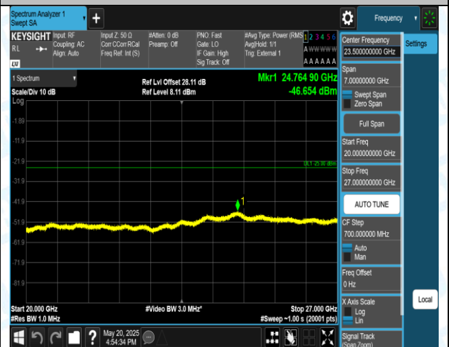
41(2555-2655)-20MHz-QPSK-40690-1RB#0-20000~27000-PASS
