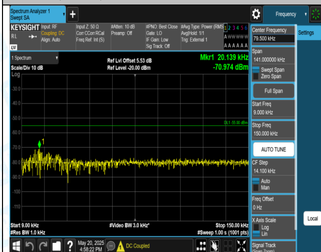
41(2555-2655)-20MHz-QPSK-41140-1RB#0-0.009~0.15-PASS
