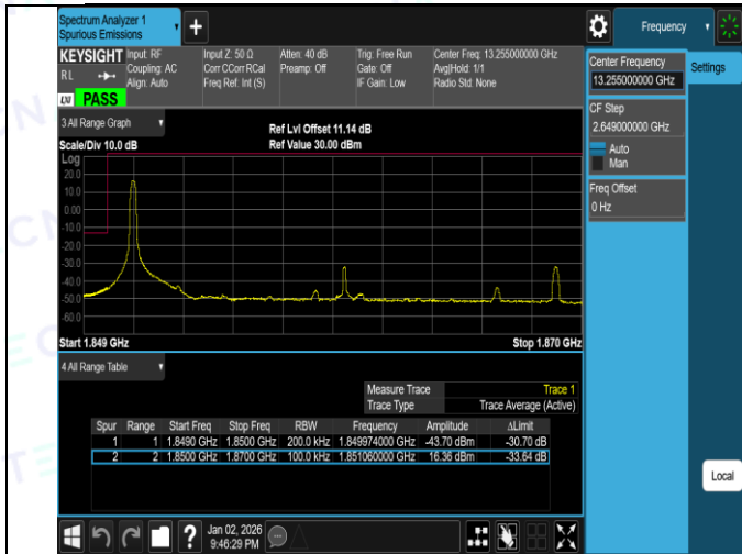
Band2-20MHz-16QAM-18700-100RB#0-PASS
