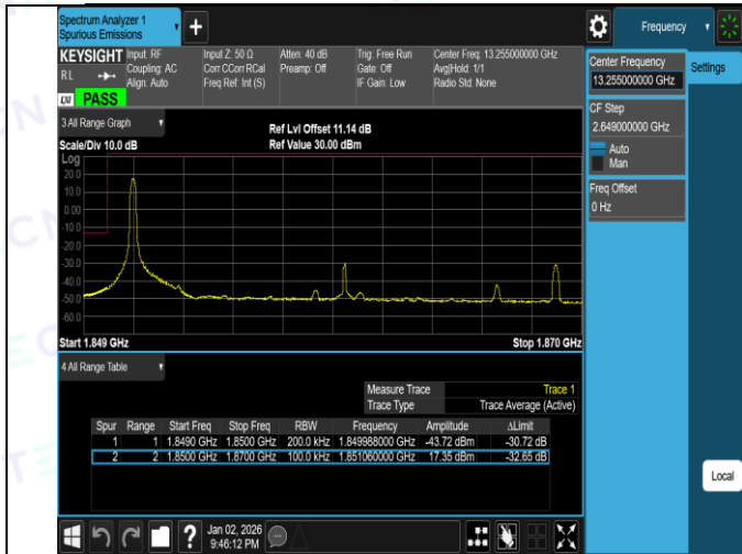
Band2-20MHz-QPSK-18700-100RB#0-PASS
