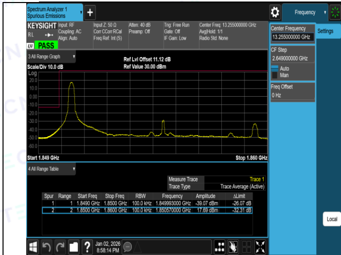
Band2-10MHz-QPSK-18650-50RB#0-PASS
