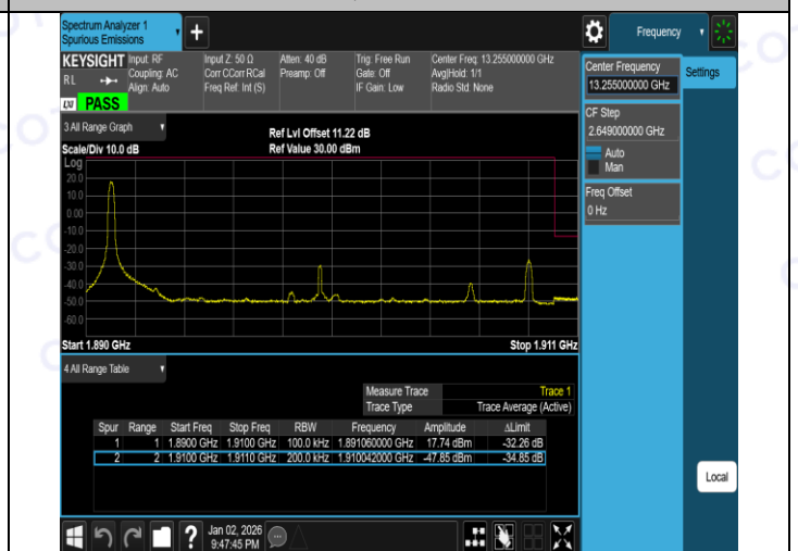
Band2-20MHz-QPSK-19100-100RB#0-PASS
