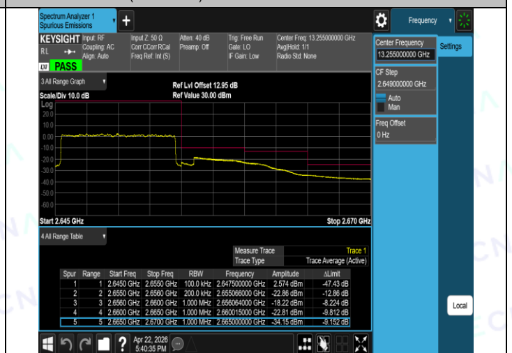
Band41(2535-2655)-10MHz-16QAM-40090-1RB#49-PASS
