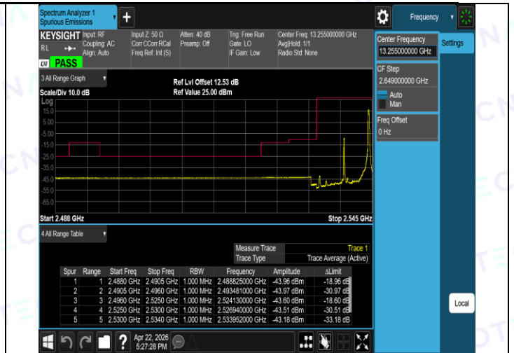
Band41(2535-2655)-10MHz-QPSK-41190-1RB#0-PASS
