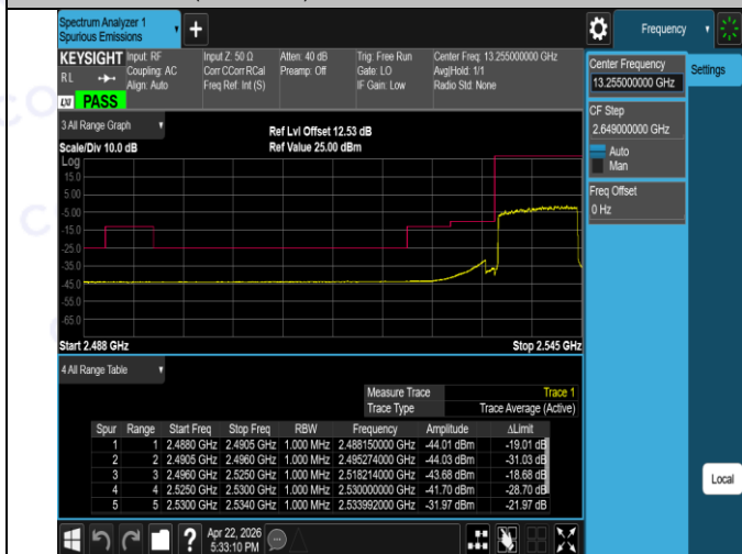
Band41(2535-2655)-10MHz-16QAM-41190-1RB#49-PASS
