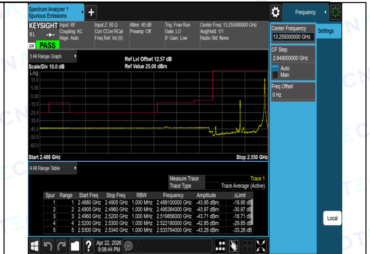
Band41(2535-2655)-15MHz-QPSK-41165-1RB#0-PASS
