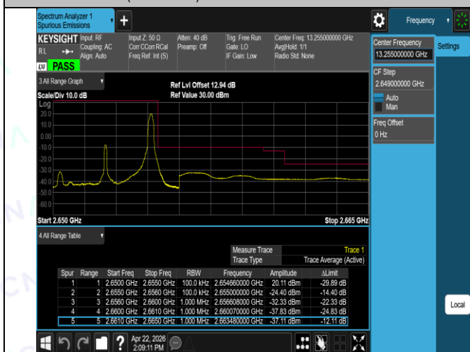
Band41(2535-2655)-10MHz-QPSK-40090-1RB#0-PASS
