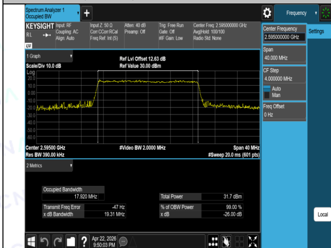
Band41(2535-2655)-20MHz-16QAM-40640-100RB#0-PASS
