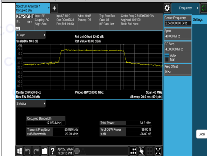
Band41(2535-2655)-20MHz-16QAM-40640-100RB#0-PASS
