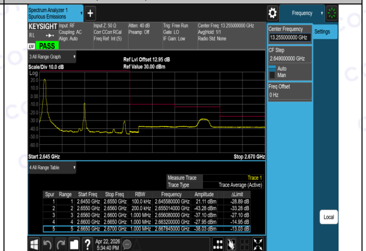
Band41(2535-2655)-10MHz-QPSK-41190-50RB#0-PASS
