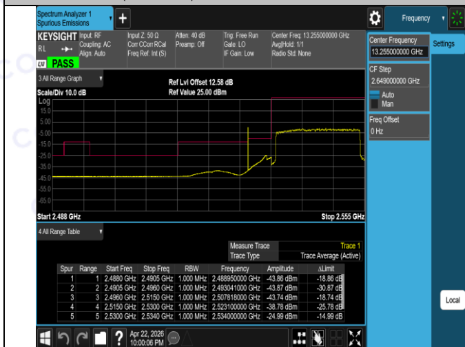
Band41(2535-2655)-20MHz-QPSK-41140-1RB#99-PASS
