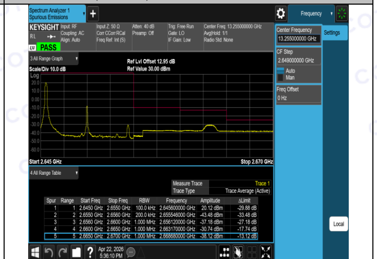
Band41(2535-2655)-10MHz-16QAM-41190-50RB#0-PASS
