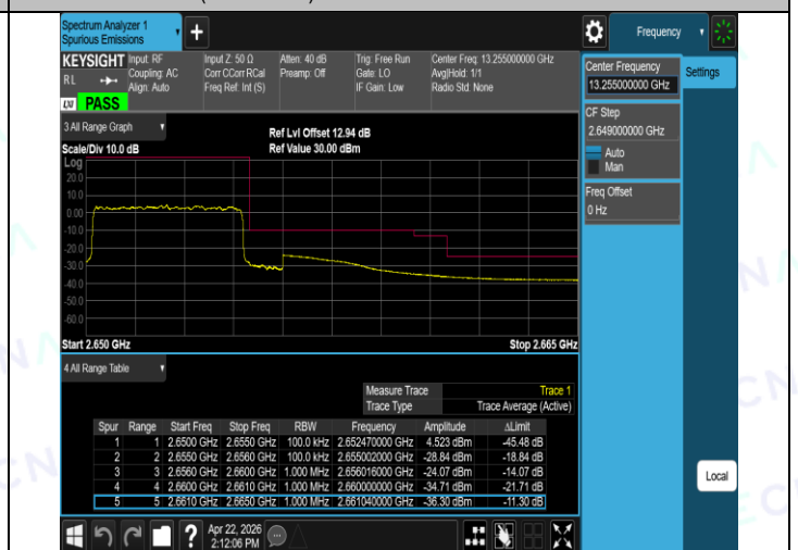
Band41(2535-2655)-10MHz-QPSK-40090-1RB#49-PASS
