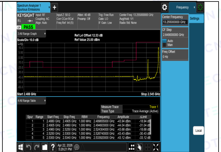
Band41(2535-2655)-10MHz-16QAM-41190-1RB#0-PASS
