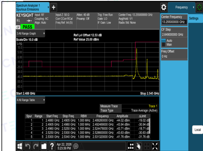
Band41(2535-2655)-10MHz-QPSK-40090-50RB#0-PASS
