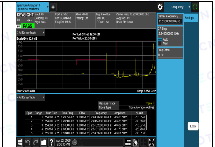
Band41(2535-2655)-20MHz-QPSK-41140-1RB#0-PASS
