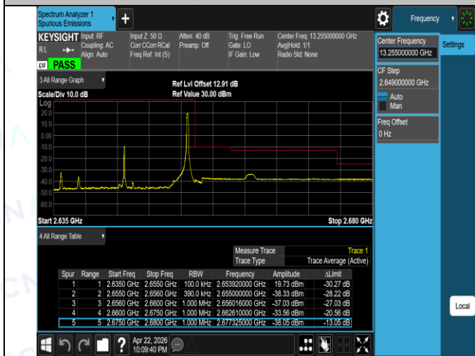
Band41(2535-2655)-20MHz-16QAM-41140-1RB#99-PASS
