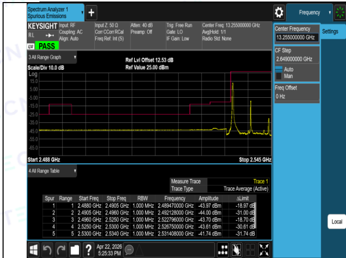
Band41(2535-2655)-10MHz-16QAM-40090-50RB#0-PASS
